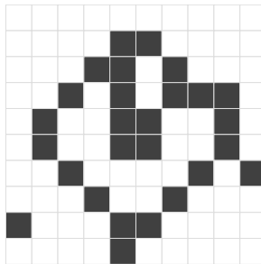
x_{t_1}
