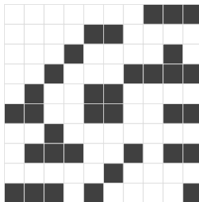
x_{t_2}
