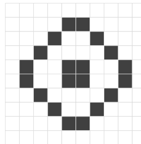
x_0 生成
