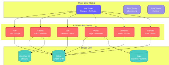
Fig. 2. Arquitectura del sistema SmartPyME: cliente móvil Flutter, API REST con Bun/Hono, y capa de almacenamiento.
