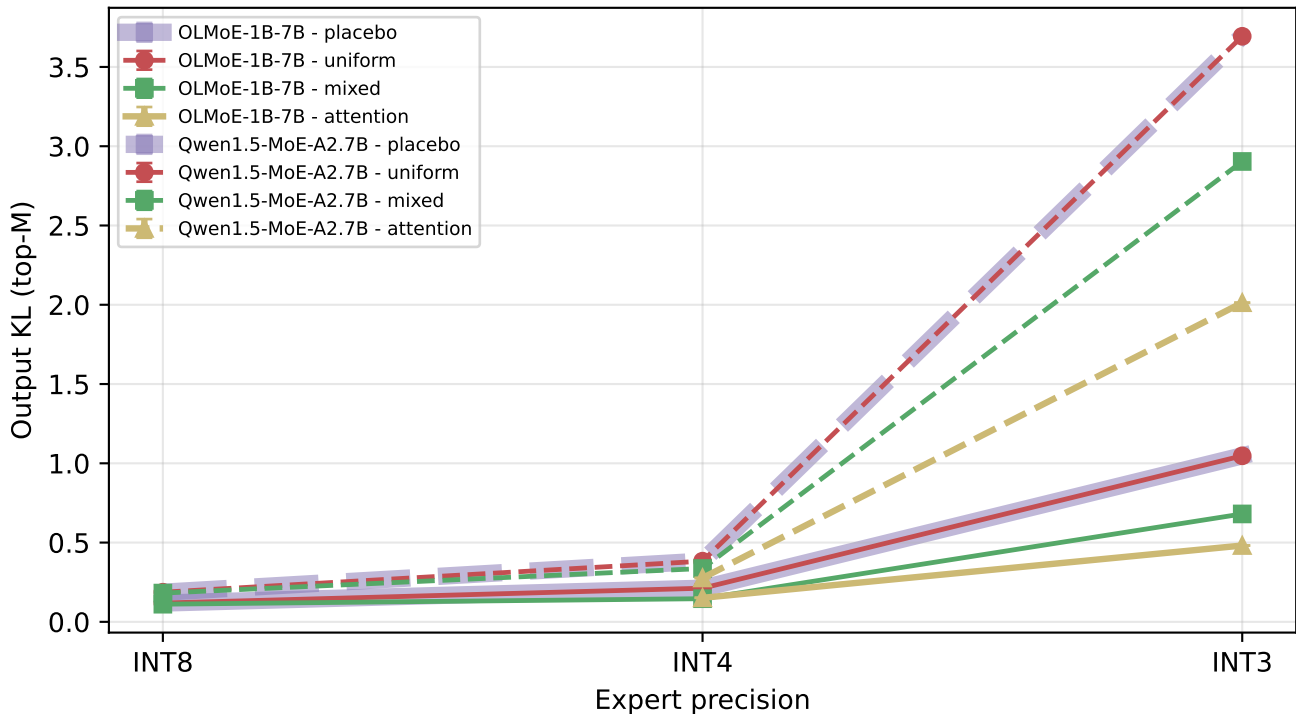
Output KL (top-M)
