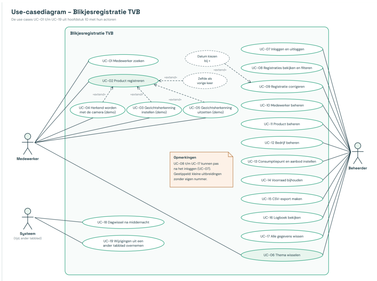
Figuur: use-casediagram met de actoren Medewerker, Beheerder en Systeem en de use cases UC-01 tot en met UC-19 uit dit hoofdstuk. UC-03, UC-04 en UC-05 zijn getekend als «extend» van UC-02.
