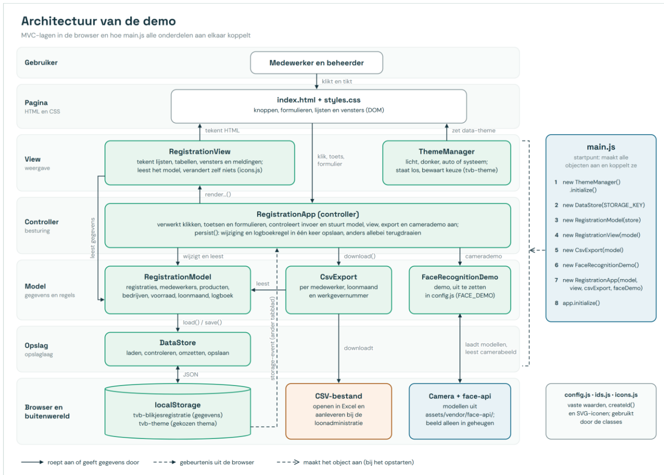
Figuur: architectuur van de demo. View, controller en model in de browser; DataStore is de enige class die de gegevens in localStorage leest en schrijft (ThemeManager bewaart daar alleen de thema-instelling); CsvExport, ThemeManager en FaceRecognitionDemo staan ernaast.
