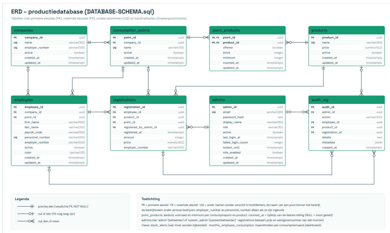
Figuur: ERD van het productieschema (DATABASE-SCHEMA.sql) met primaire en vreemde sleutels en kardinaliteiten.
