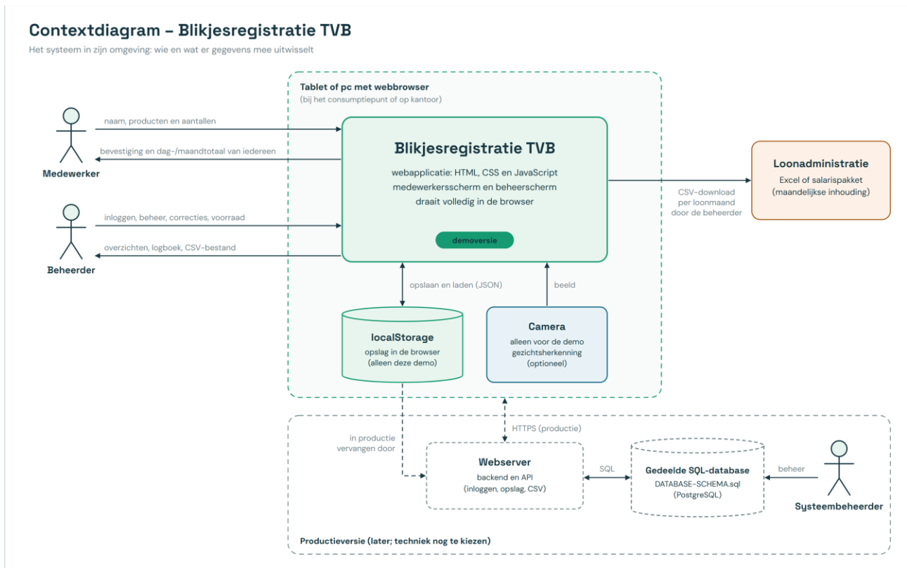
Figuur: contextdiagram. Het systeem met de medewerker, de beheerder, de tablet met browser, de opslag in localStorage, het CSV-bestand voor de loonadministratie en (in productie) de server met database.
