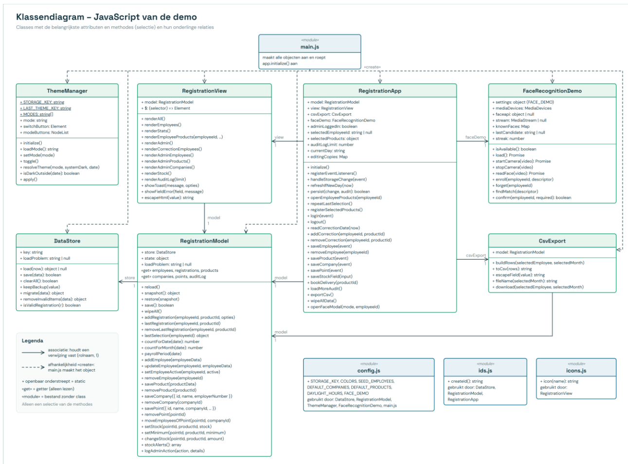
Figuur: klassendiagram van de JavaScript met de belangrijkste attributen, methodes en relaties.
