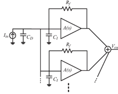
圖二 用於增強頻寬的 TIA 結構
