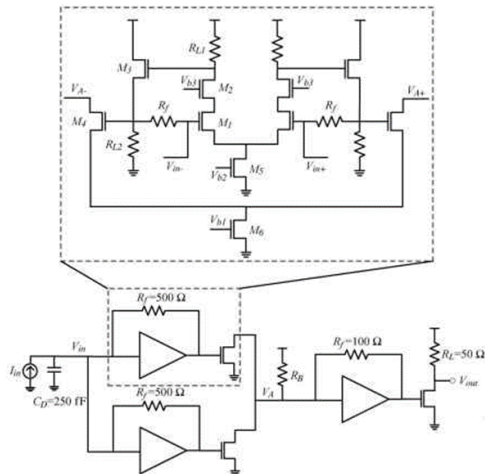
圖三 差動 TIA 結構圖
