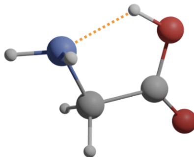
\text{OH} \cdots \text{NH}_2 motif
