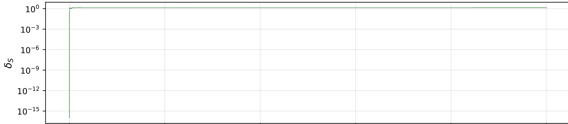
Kekekalan norma spin
