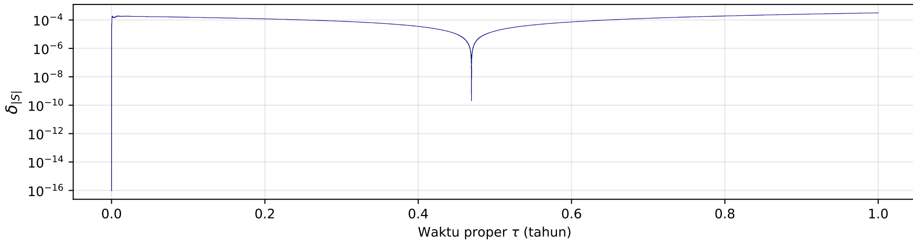
Kekekalan norma spin
