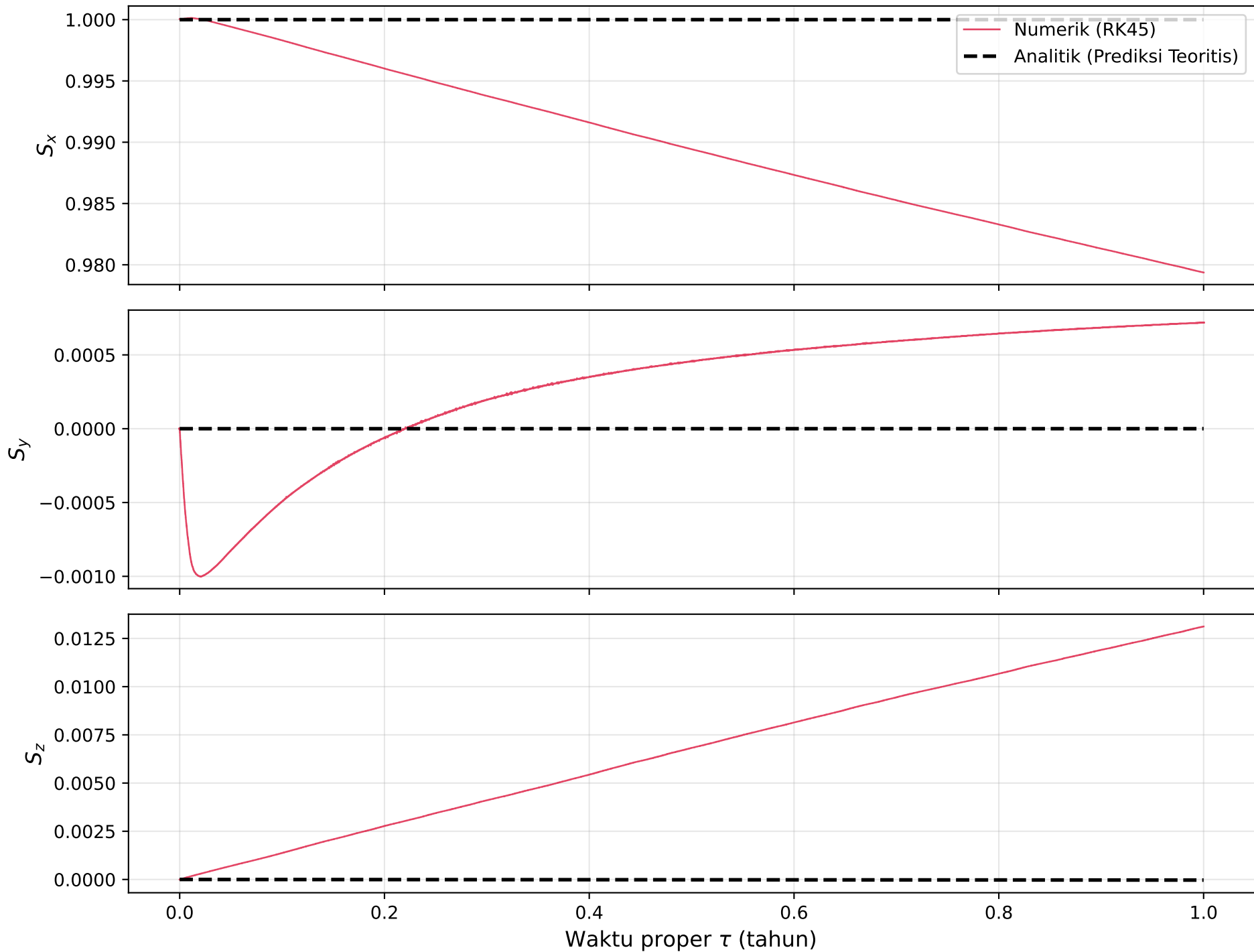
Kegagalan RK45: Numerik vs Analitik (1 Tahun)
