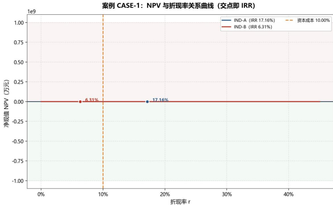
图 3-4 CASE-1 的 NPV—折现率曲线：与横轴交点即 IRR
