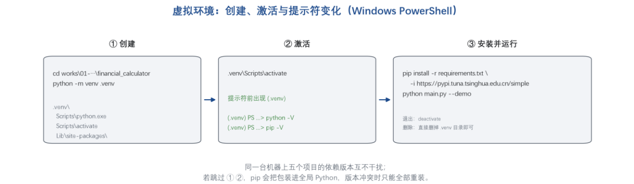
图 1-14 虚拟环境的创建、激活与提示符变化 本手册自绘
