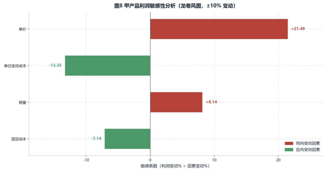
图 4-7 利润敏感性龙卷风图：四因素冲击幅度排序
