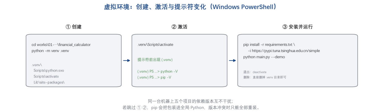
图 1-14 虚拟环境的创建、激活与提示符变化
