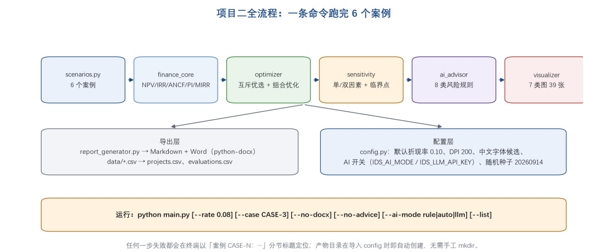
图 3-1 项目二的模块流水线与命令行开关
