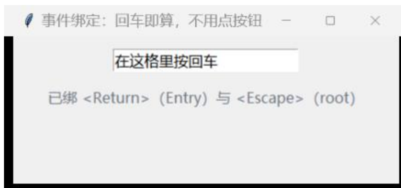
图 I-6 <Return> 绑在 Entry 上、<Escape> 绑在 root 上
