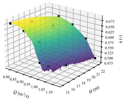
LHS
