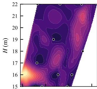
LHS
