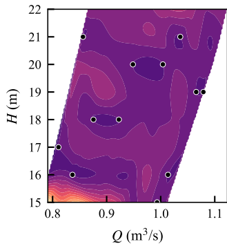
LHS
