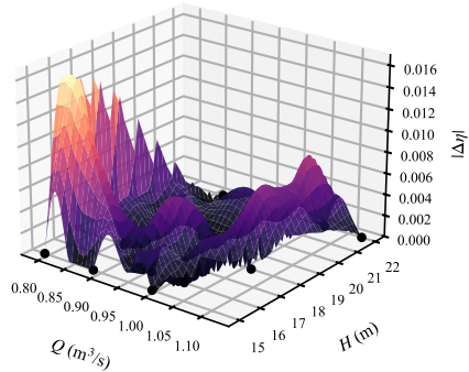
LHS
