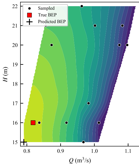
ALC (MAE=0.0026)
