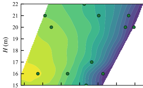
ALC ( n=12 )
