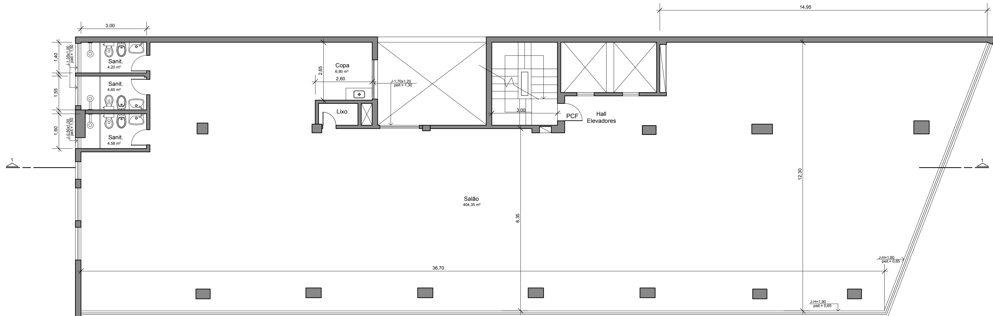
7º Pavimento
