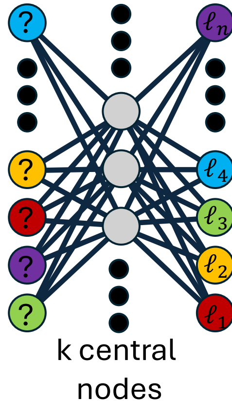
(d) Two-Radius (general k )
