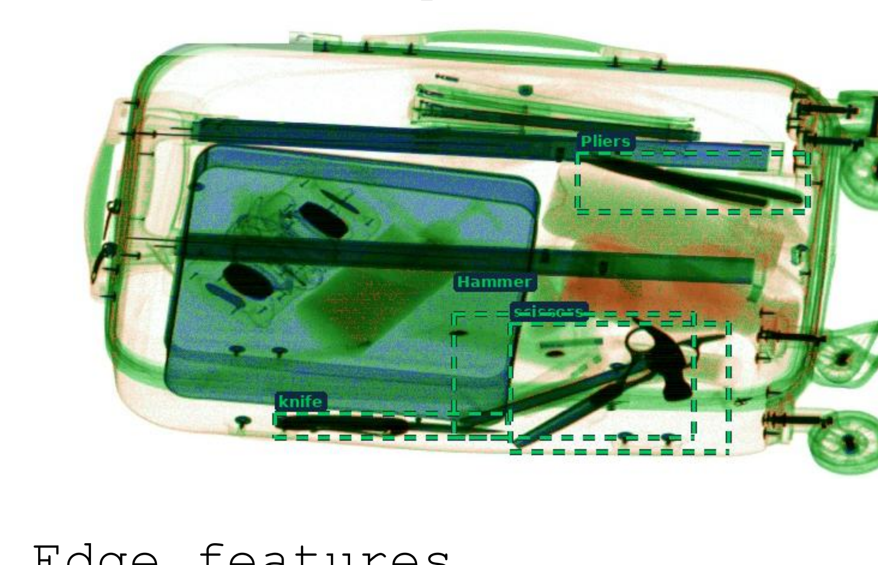
Input
