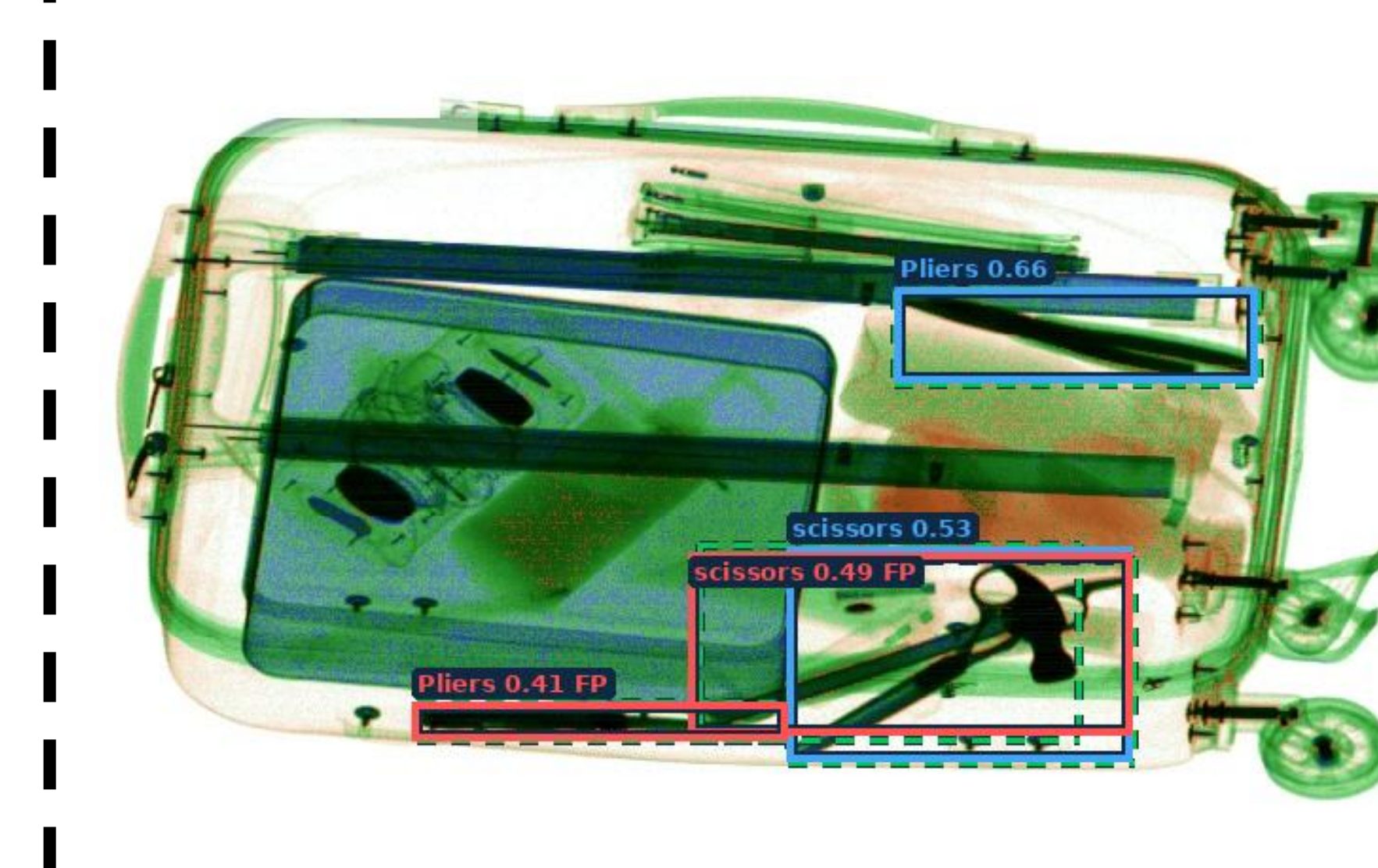
Baseline
