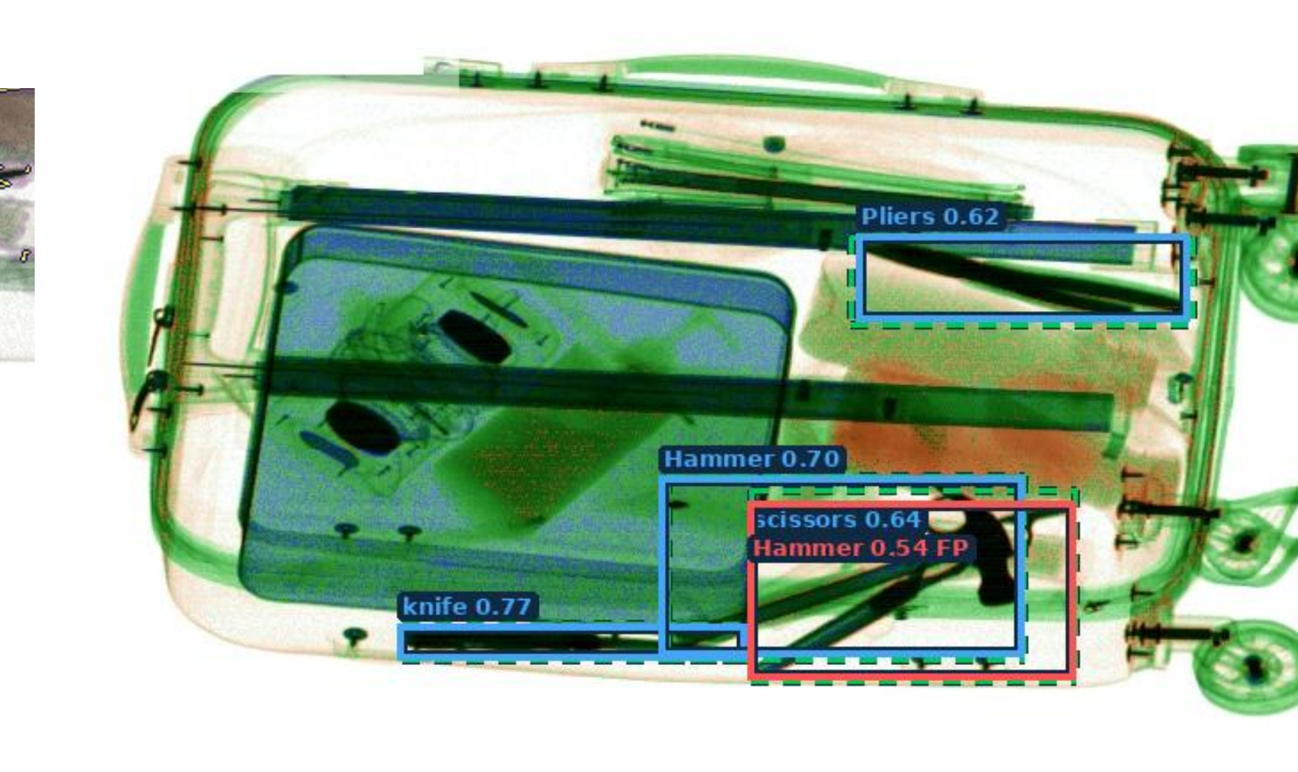
DERA
