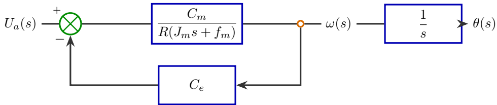
等效简化形式
