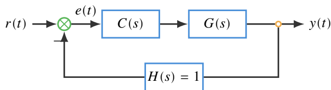
图 1-1-7. 单位负反馈闭环系统
