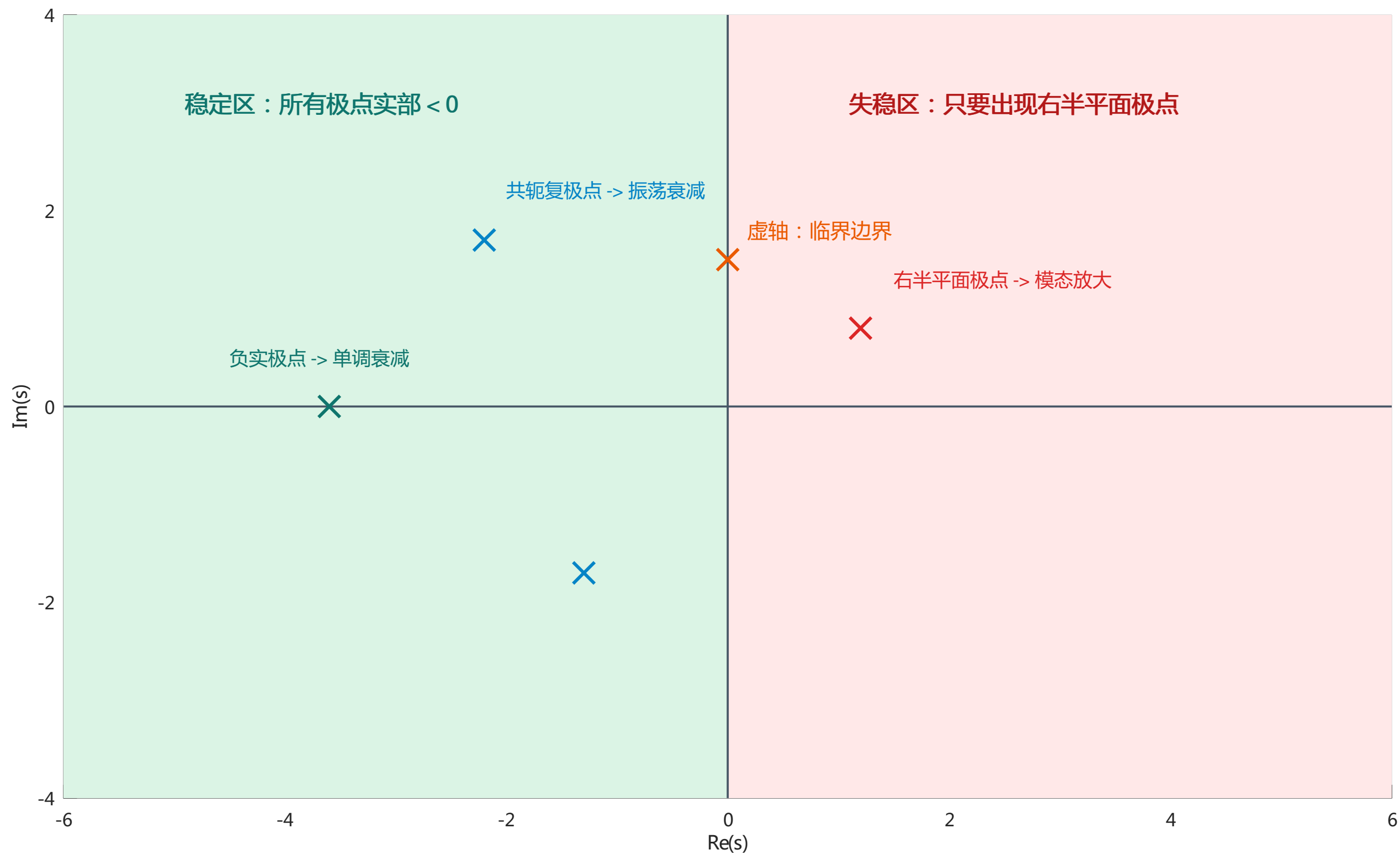
闭环极点在复平面中的位置先决定稳定底线
