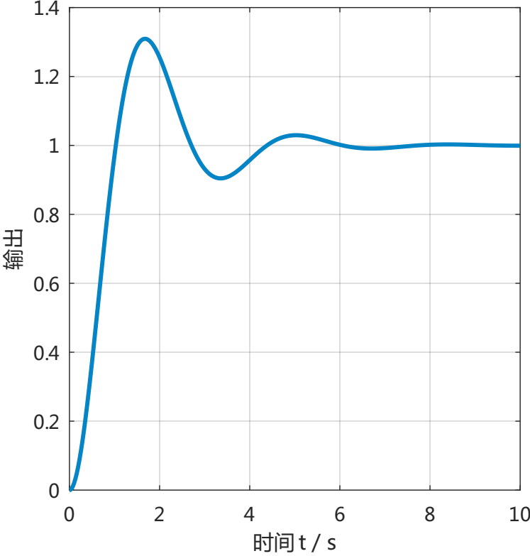
响应 B：振荡衰减
