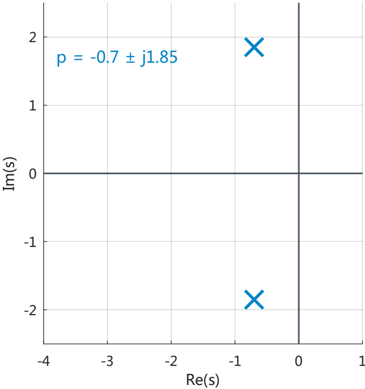
极点 B：左半平面共轭极点
