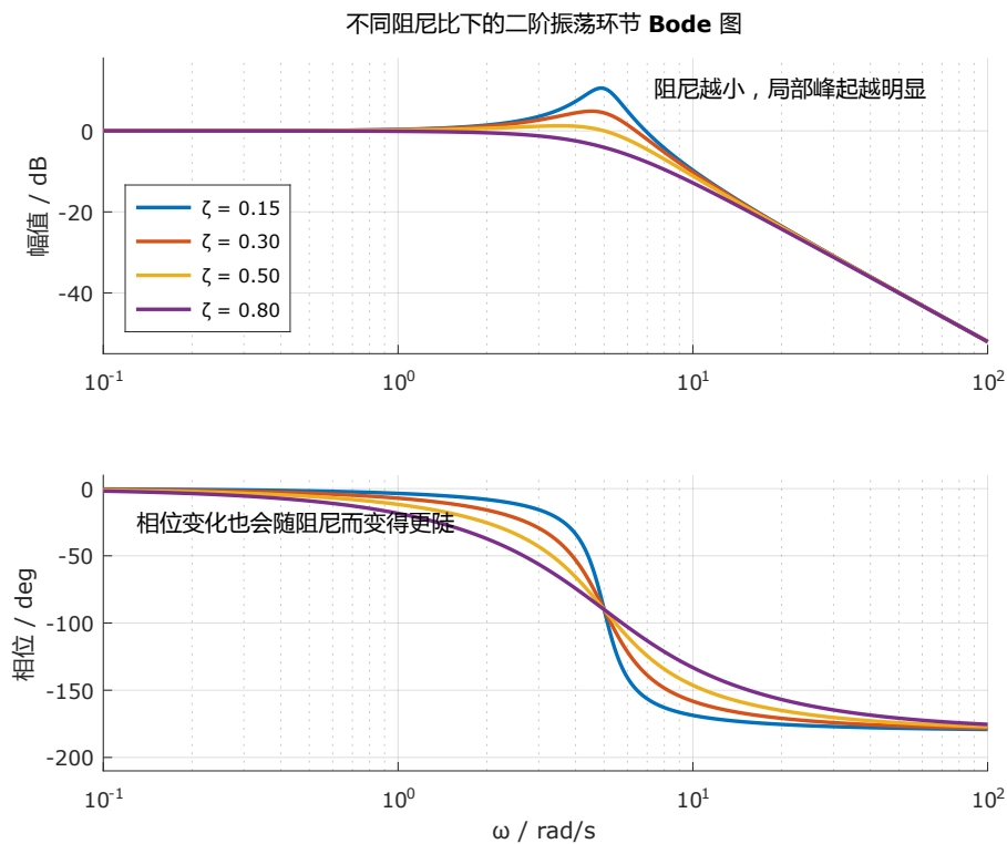
图 8. 二阶振荡环节阻尼变化下的 Bode 图
