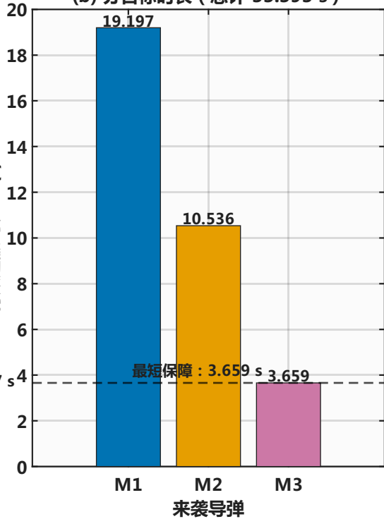
(b) 分目标时长 (总计 33.393 s)
