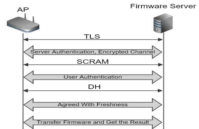
[그림 4-1] 경북대 이임영 교수가 제안한 펌웨어 업데이트 프로토콜
