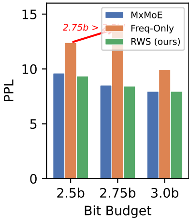
Qwen1.5-MoE
