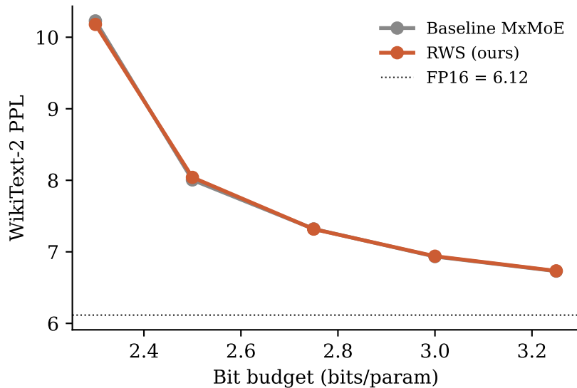
DeepSeek-MoE-16B (RHI=1.56)
