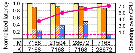
(d) MTV in GPT-J 30B.
