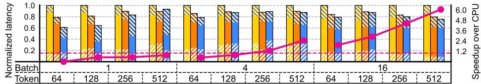
(c) MMTV in GPT-J 30B.
