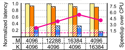
(b) MTV in GPT-J 6B.
