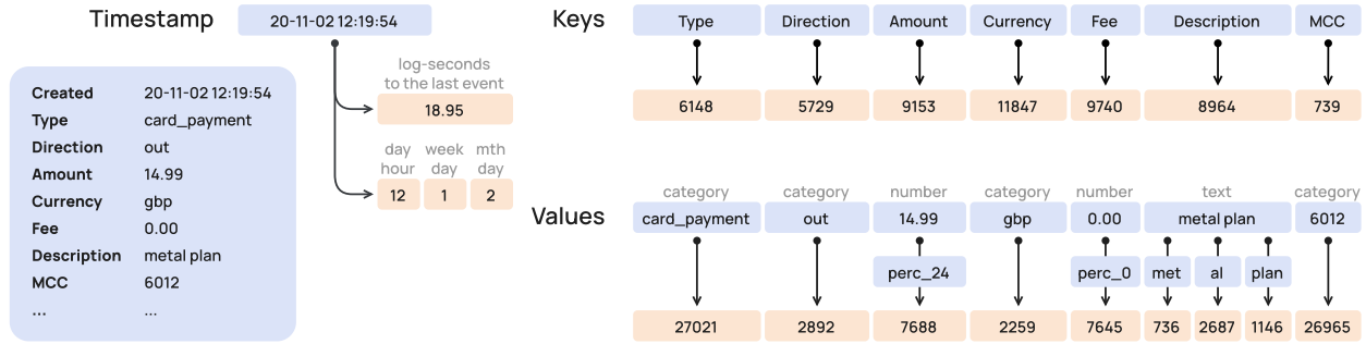
그림 3: 토큰화 개요. 원시 이벤트 레코드는 시간 좌표, 의미 타입(키), 값으로 분해된다. 키는 항상 하나의 토큰으로 표현되고, 값은 타입별 토큰화를 따른다 — 수치값은 백분위 버킷으로, 범주값은 하나의 토큰으로, 텍스트 값은 서브워드 토큰들로 분해된다. 따라서 어떤 키는 여러 개의 값 토큰으로 펼쳐지기도 한다(예: Description → met , al , plan ). 시간은 직전 이벤트까지의 로그-초(log-seconds)와, 타임스탬프에서 유도된 달력·시간 피쳐로 함께 인코딩된다. 프로필 상태는 이벤트 레코드와 비슷하게 인코딩된다.
