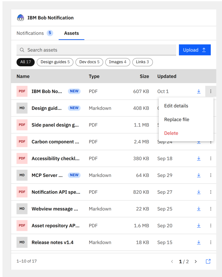
Admin — 넓은 Assets와 자료 관리 메뉴
