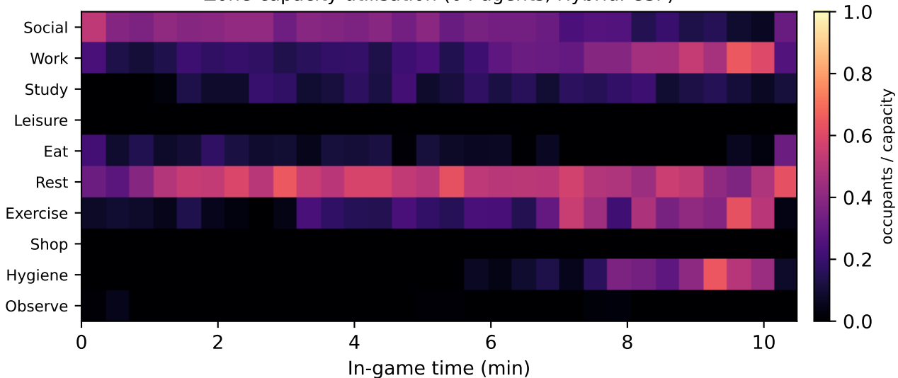
Zone-capacity utilisation (64 agents, HybridPCSP)
