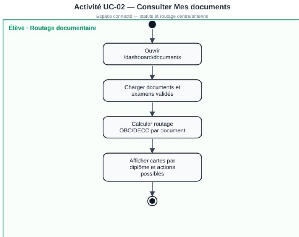
Figure 3.9 — Activité UC-02 : Mes documents
