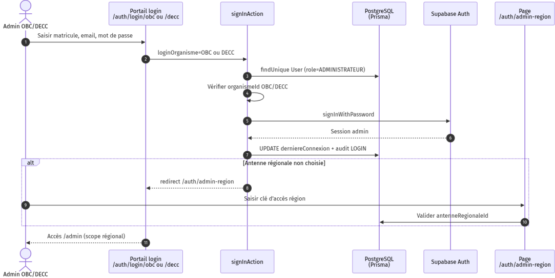
Figure 3.22 — Séquence auth admin
