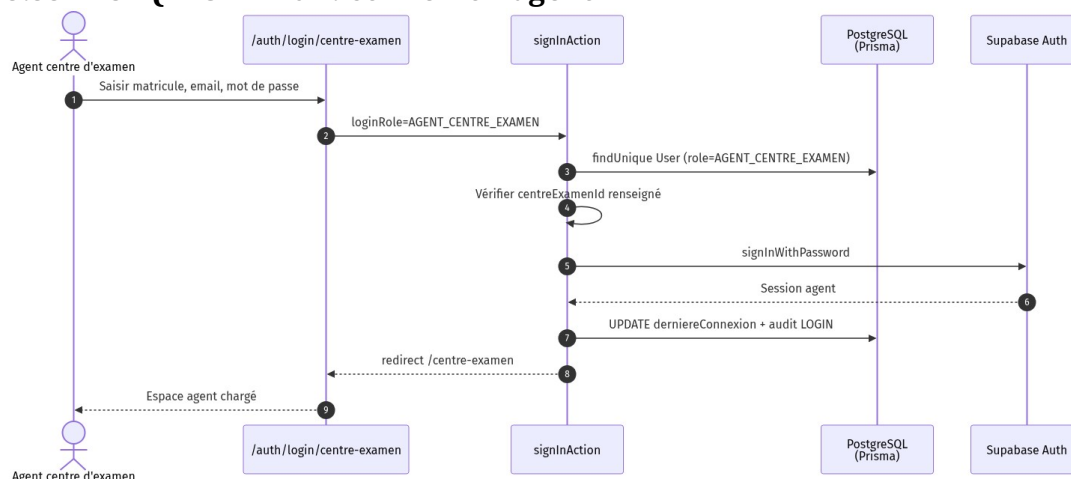
Figure 3.33 — Séquence auth agent
