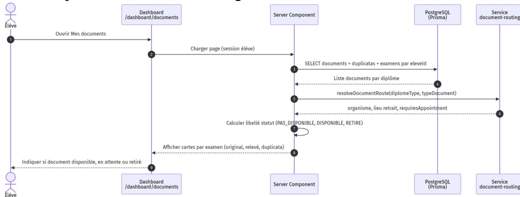
Figure 3.10 — Séquence Mes documents
