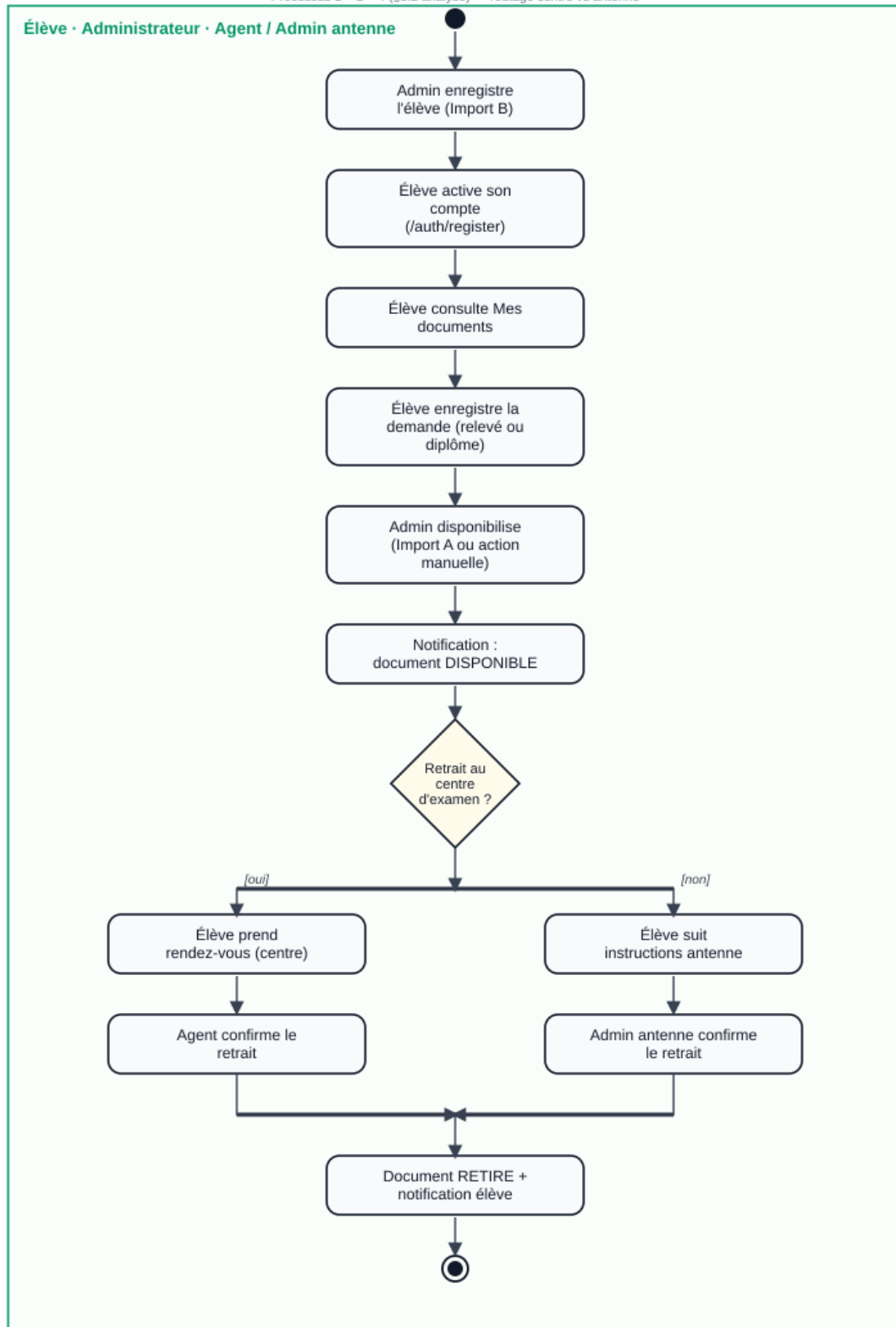
Figure 3.38 — ACT-01 parcours retrait
