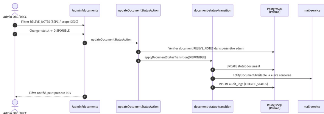
Figure 3.28 — Séquence MAJ statut
