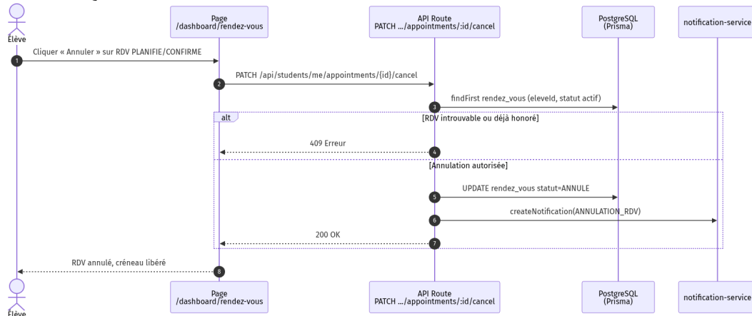
Figure 3.20 — Séquence annulation RDV
