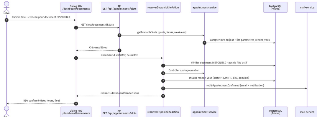
Figure 3.19 — Séquence prise RDV
