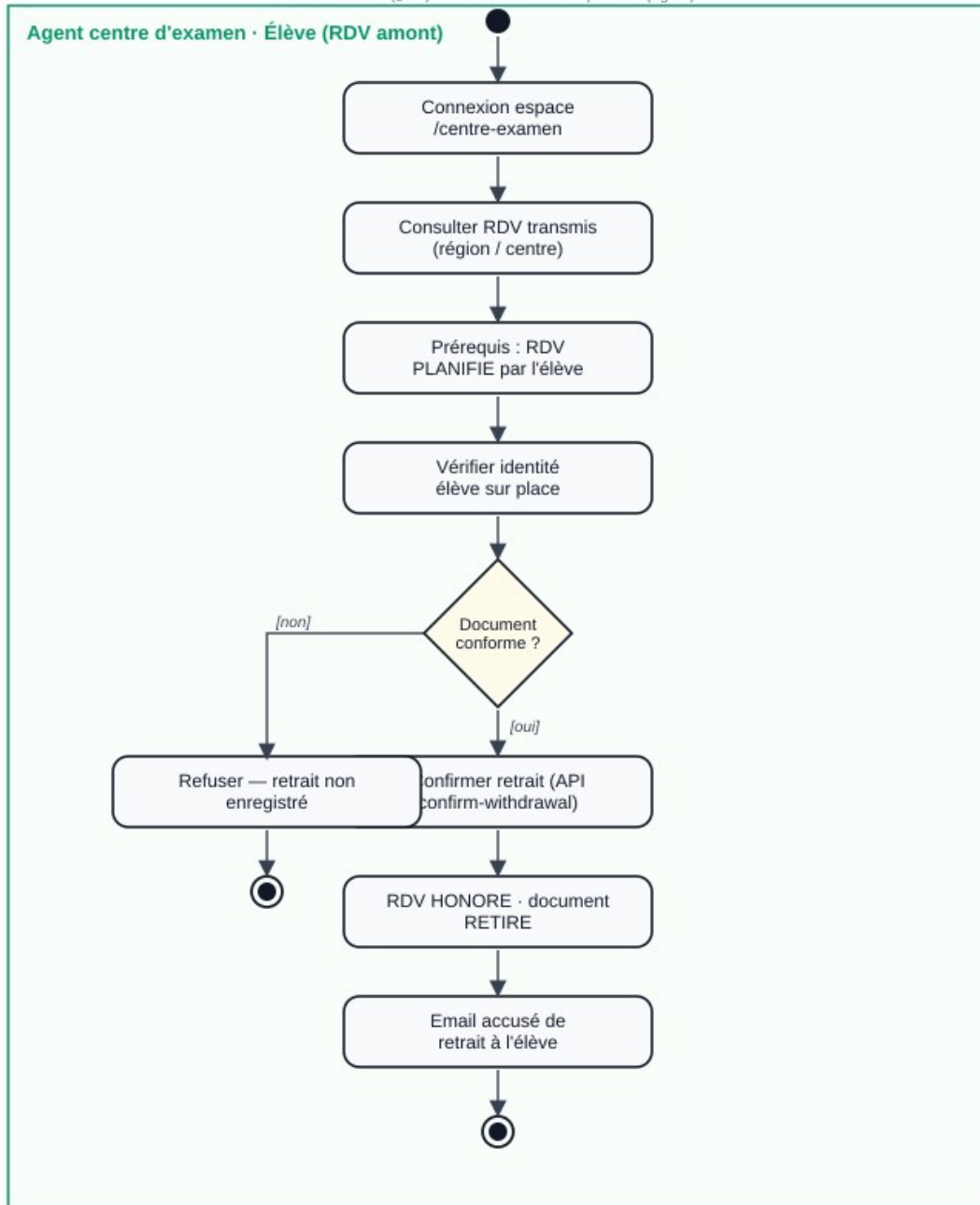
Figure 3.36 — Activité confirmation retrait
