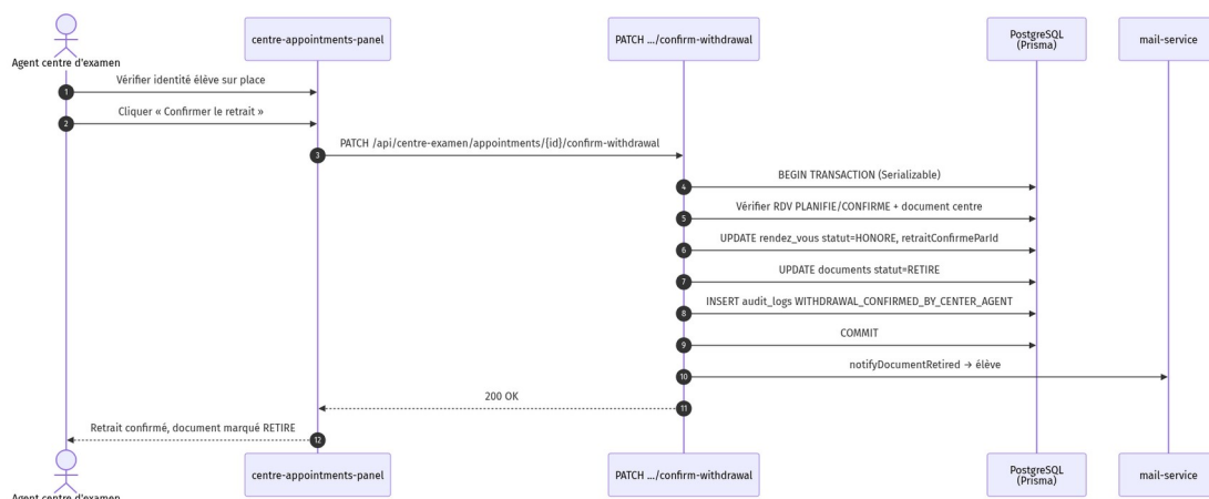
Figure 3.37 — Séquence confirmation retrait
