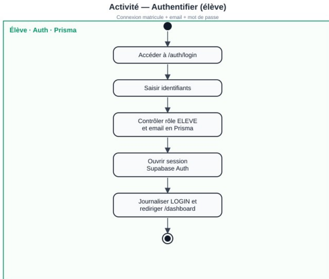
Figure 3.5 — Activité authentification élève
