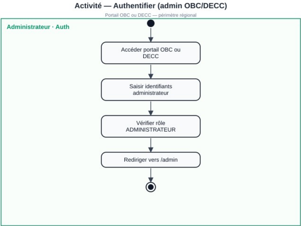
Figure 3.21 — Activité auth admin
