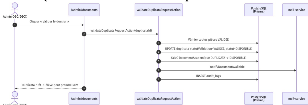
Figure 3.30 — Séquence validation duplicata
