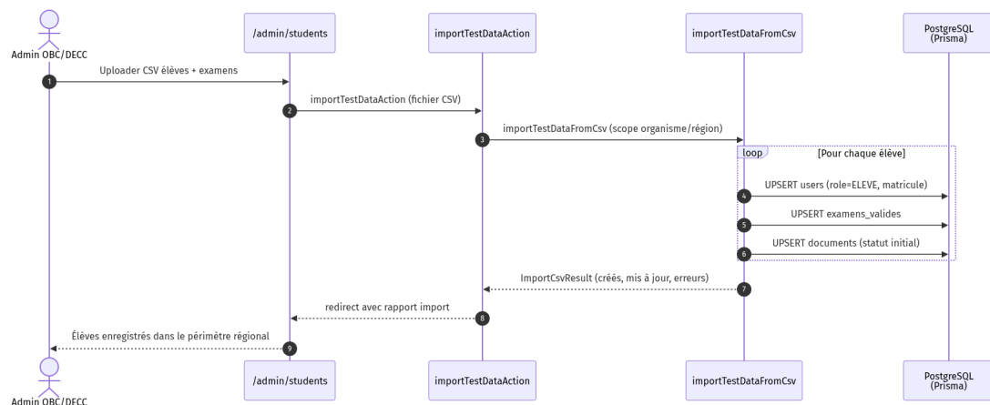
Figure 3.24 — Séquence Import B
