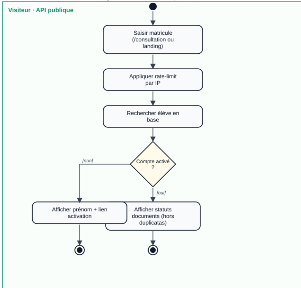
Figure 3.7 — Activité UC-03
