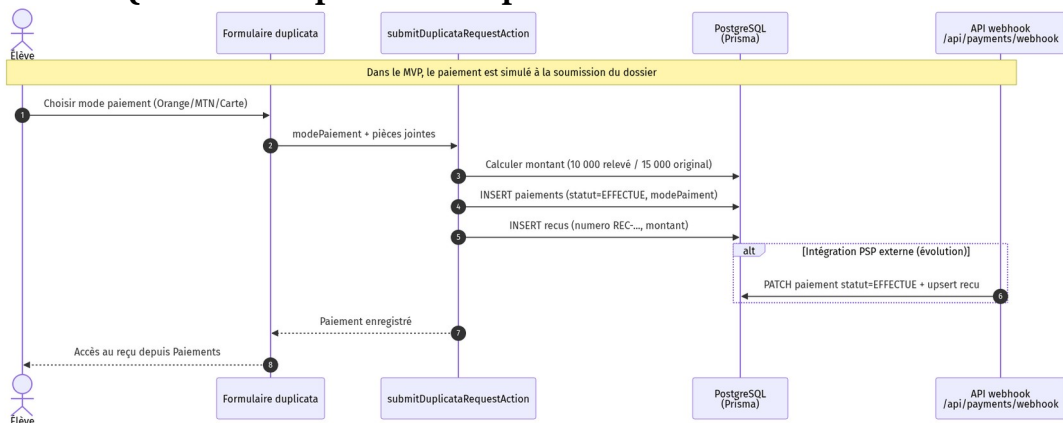
Figure 3.16 — Séquence paiement
