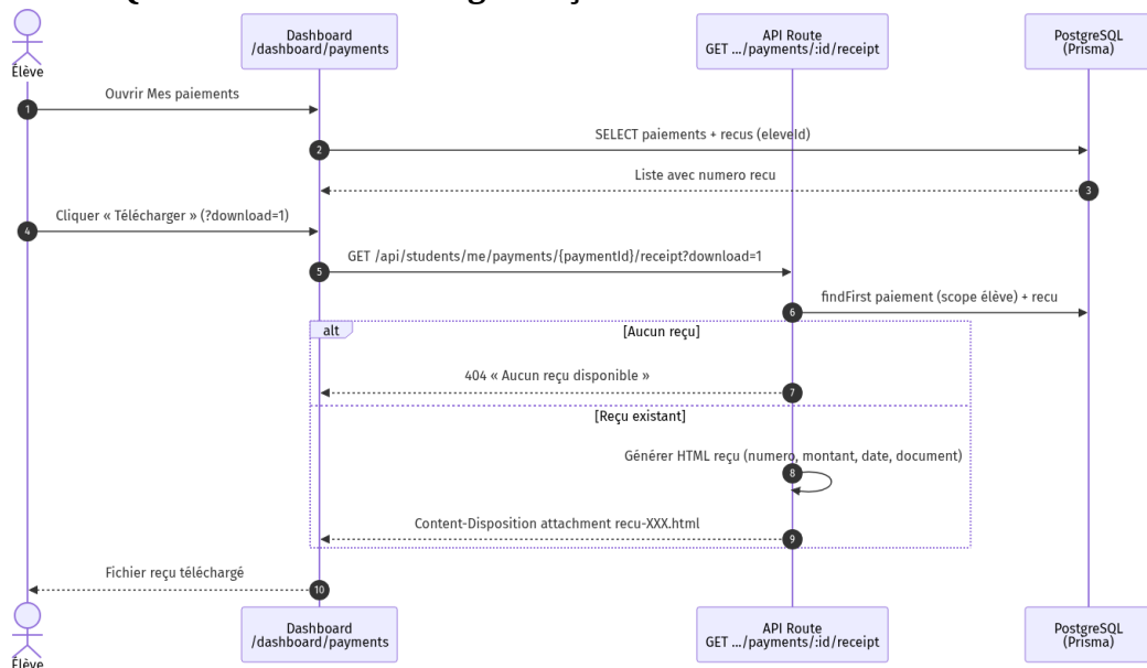
Figure 3.17 — Séquence reçu
