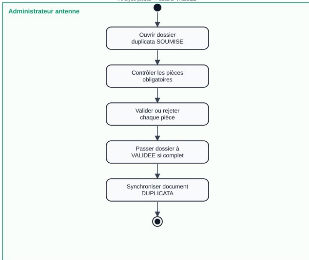
Figure 3.29 — Activité UC-10
