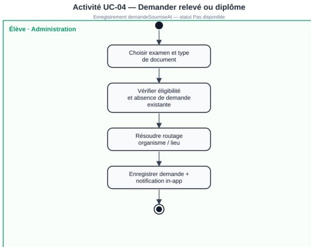
Figure 3.11 — Activité UC-04
