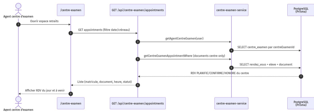
Figure 3.35 — Séquence consulter RDV
