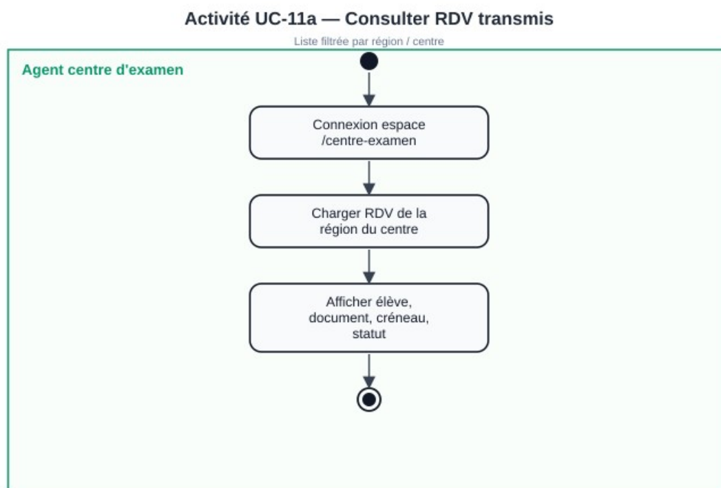
Figure 3.34 — Activité consulter RDV
