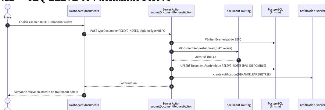
Figure 3.12 — Séquence demande relevé
