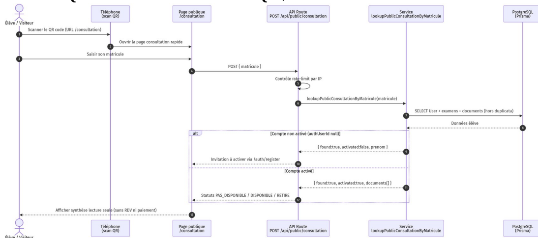
Figure 3.8 — Séquence consultation publique
