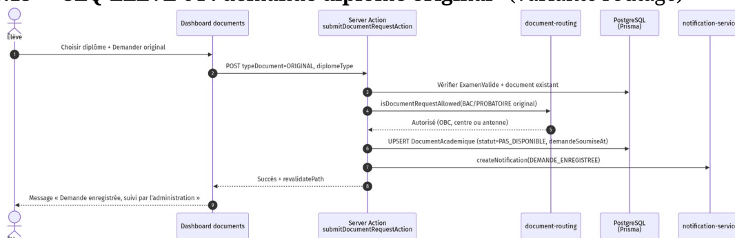
Figure 3.13 — SEQ-ELEVE-04 : demande diplôme original *(variante routage)*
