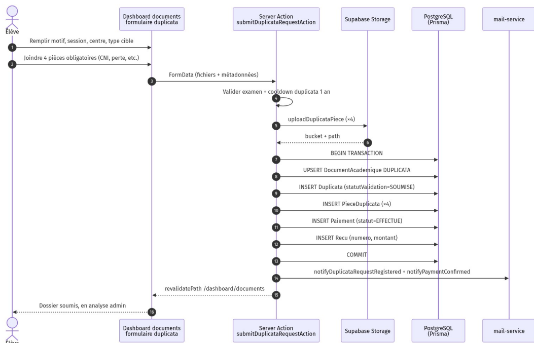
Figure 3.15 — Séquence formulaire duplicata
