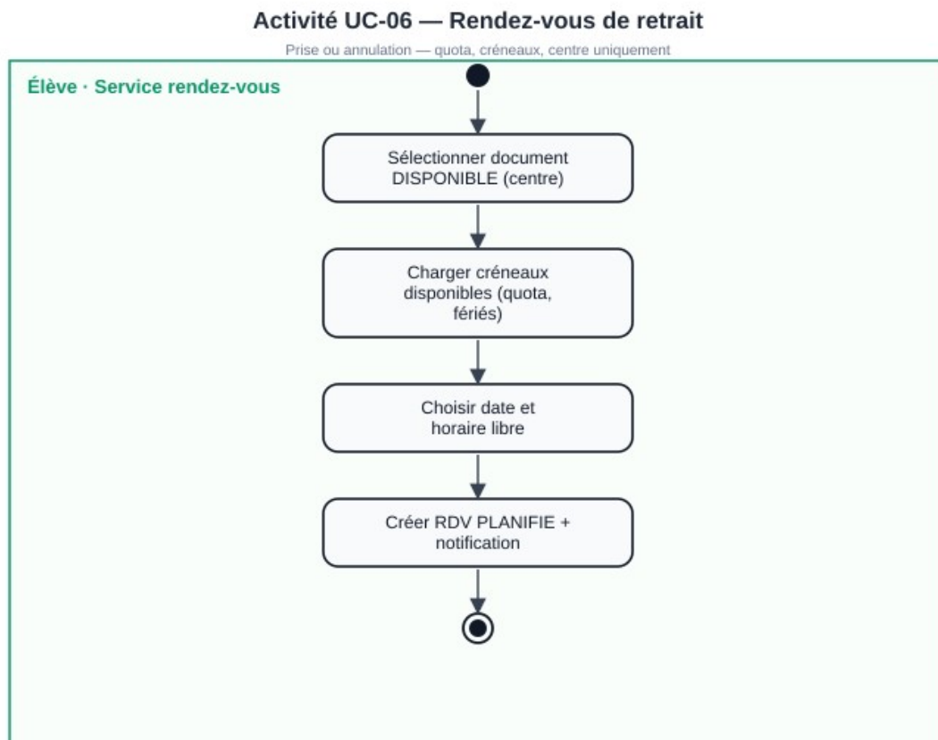
Figure 3.18 — Activité UC-06 : rendez-vous de retrait
