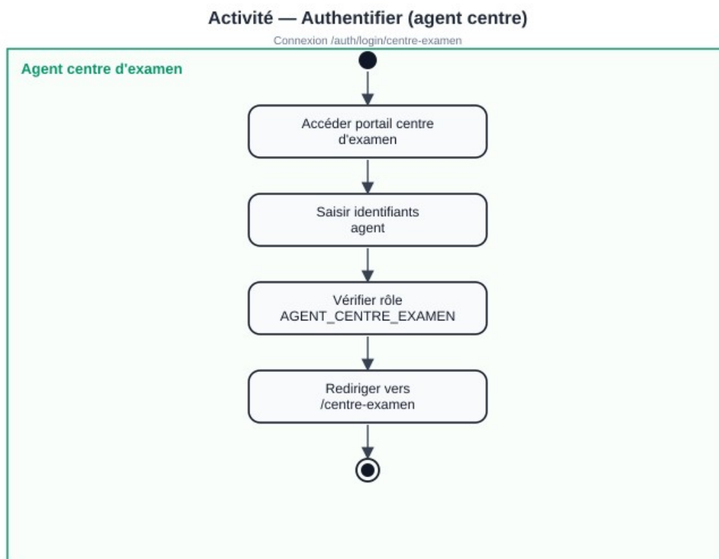
Figure 3.32 — Activité auth agent
