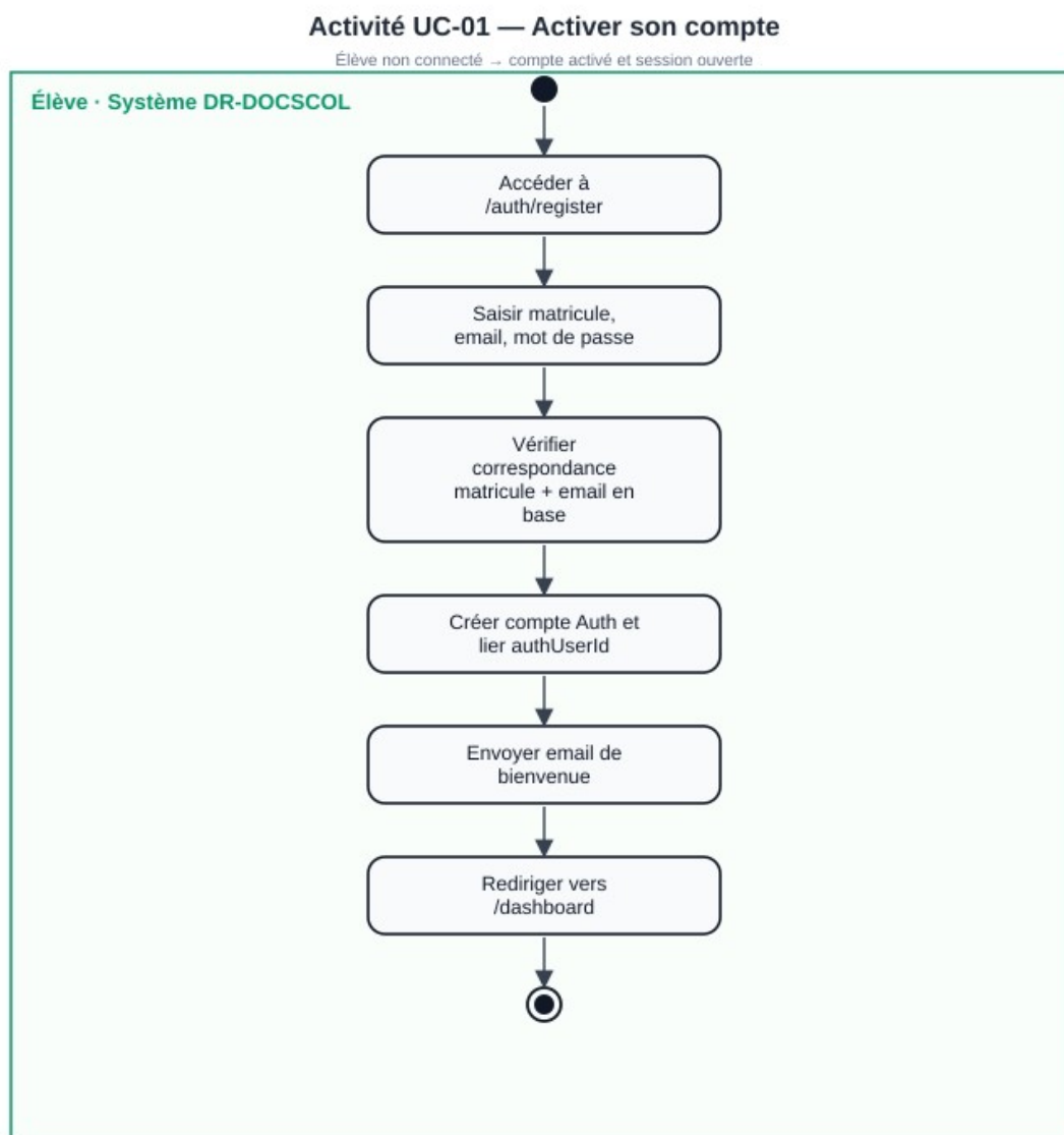
Figure 3.4 — Activité UC-01
