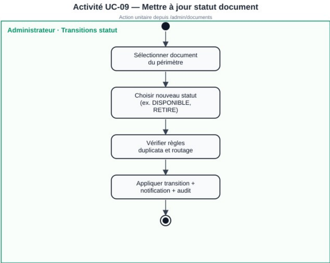
Figure 3.27 — Activité UC-09
