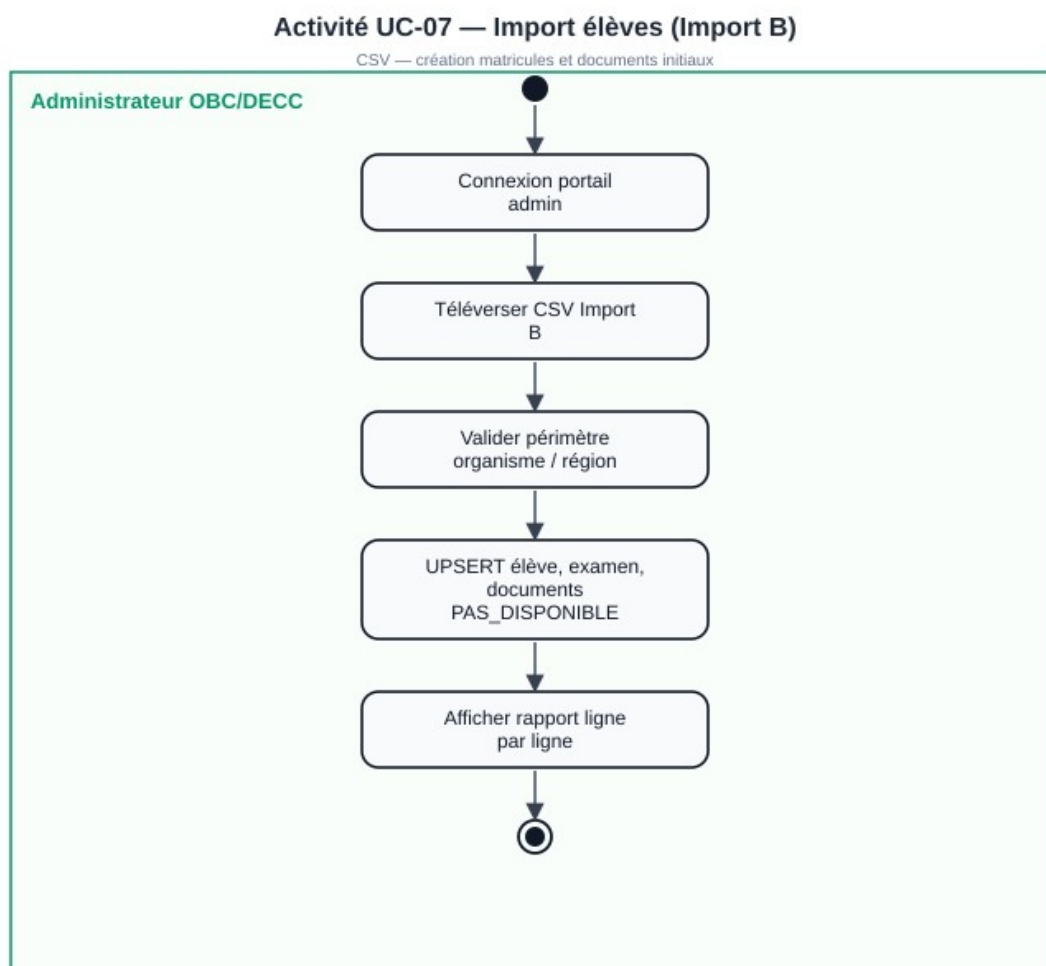
Figure 3.23 — Activité UC-07
