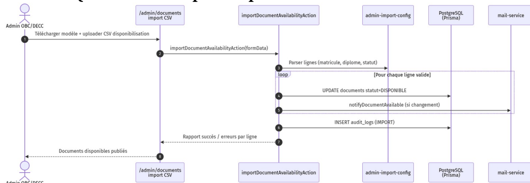
Figure 3.26 — Séquence Import A
