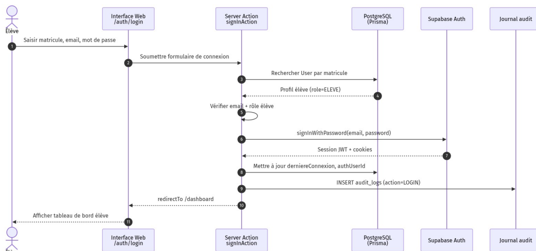
Figure 3.6 — Séquence authentification élève
