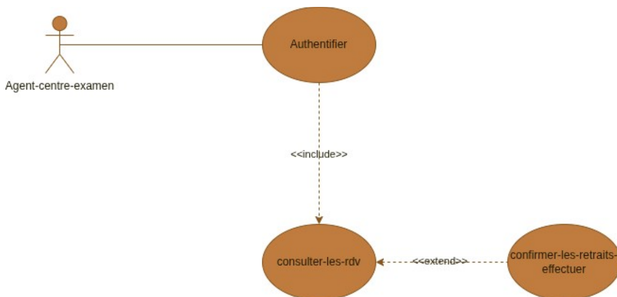
Figure 5.3 — Diagramme de cas d'utilisation — package Agent centre d'examen
