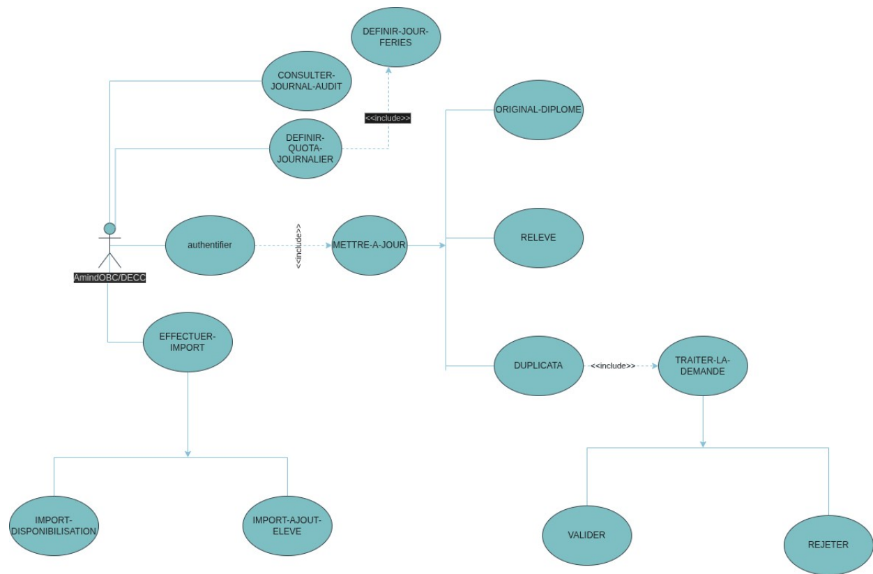
Figure 5.2 — Diagramme de cas d'utilisation — package Administrateur OBC / DECC
