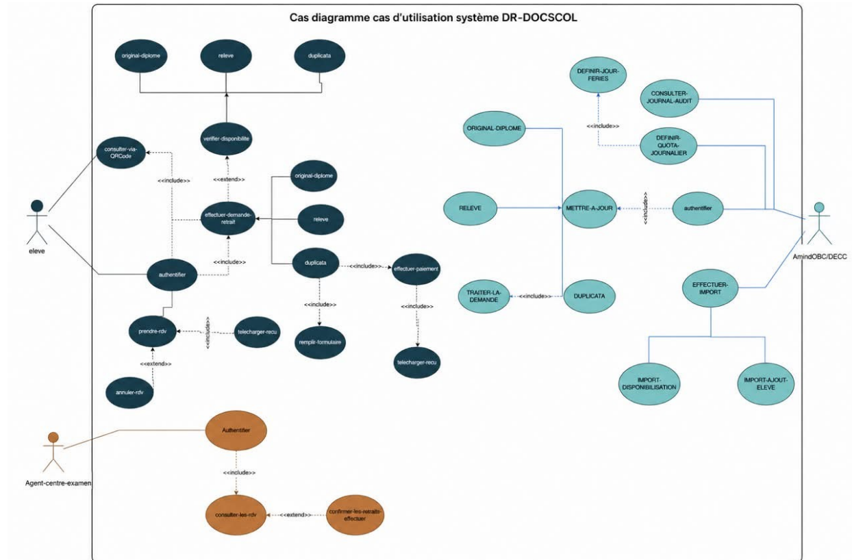
Figure 5.0 — Diagramme général des cas d'utilisation DR-DOCSCOL
