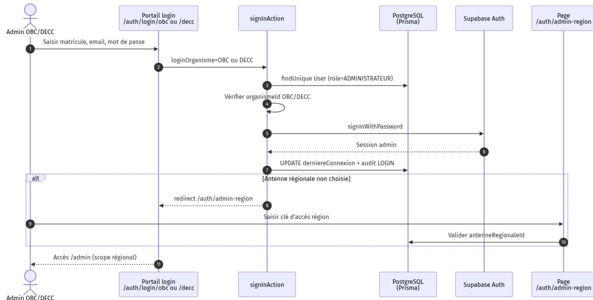
Figure 3.22 — SEQ-ADMIN-01 : connexion administrateur
