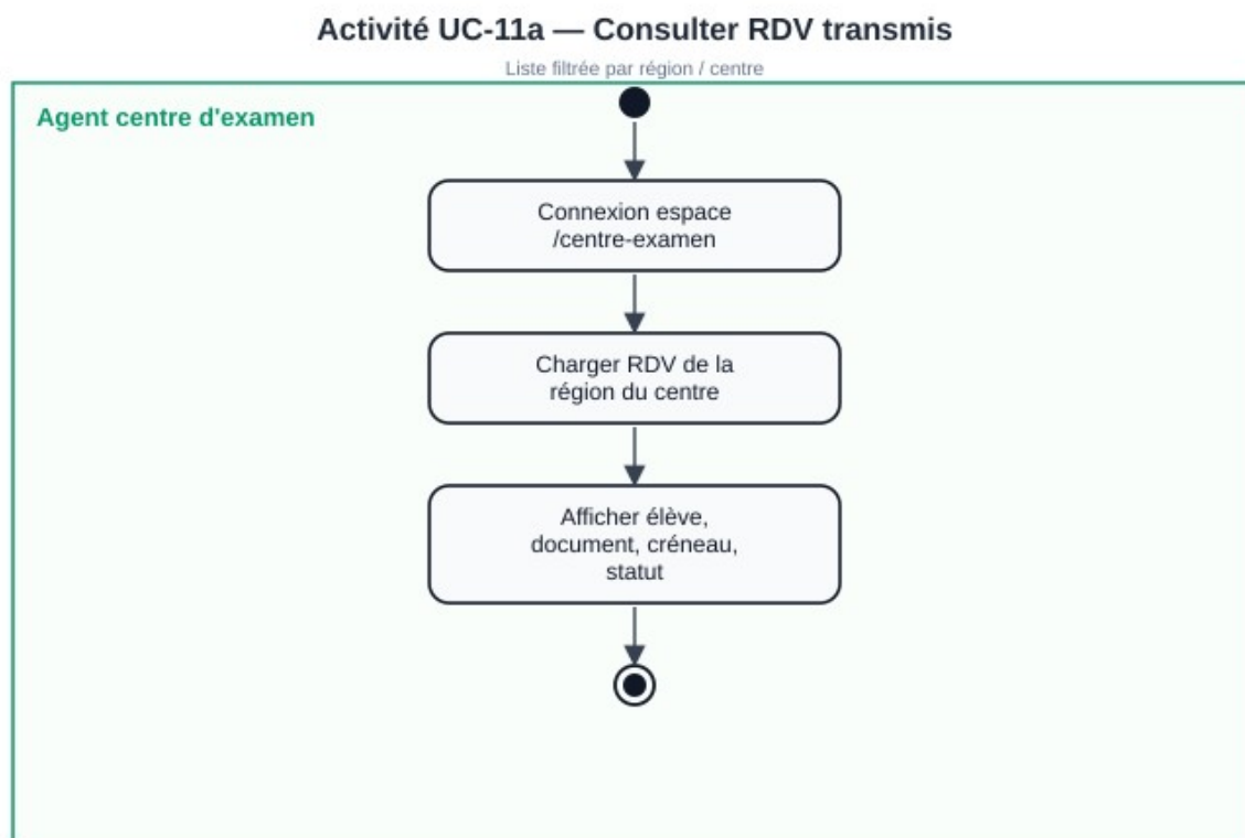
Figure 3.34 — Activité UC-11a : consulter RDV transmis
