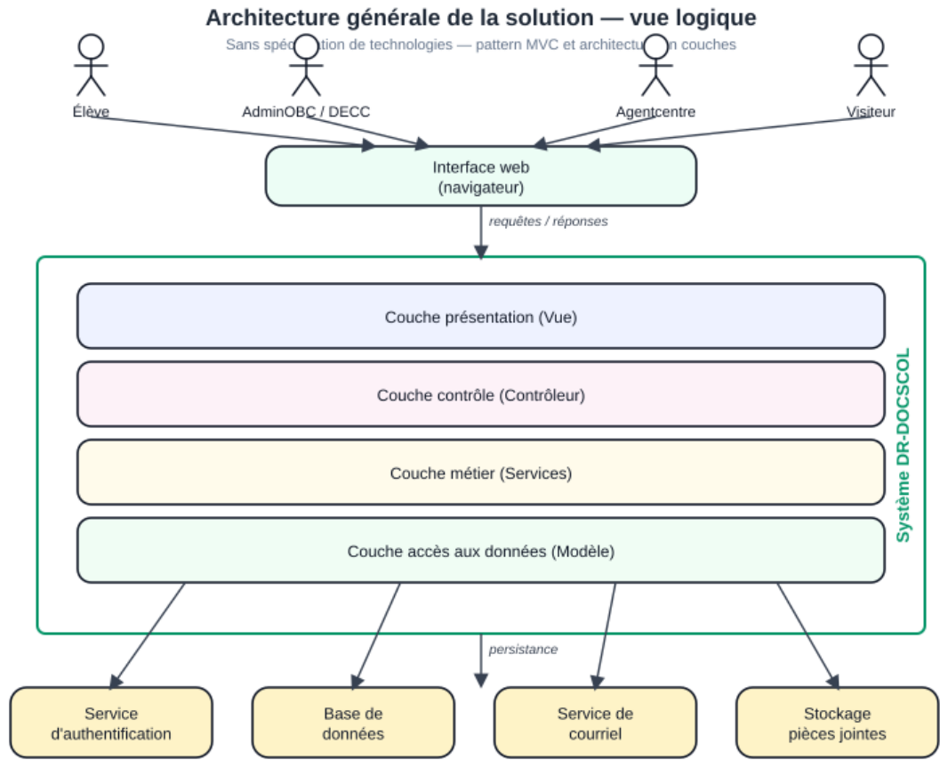
Figure 2.2 — Architecture générale de la solution (vue logique MVC)
