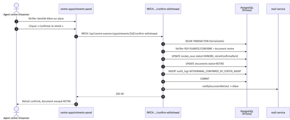
Figure 3.37 — SEQ-AGENT-03 : confirmer retrait effectué
