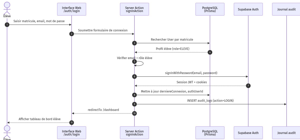
Figure 3.6 — SEQ-ELEVE-01 : connexion élève
