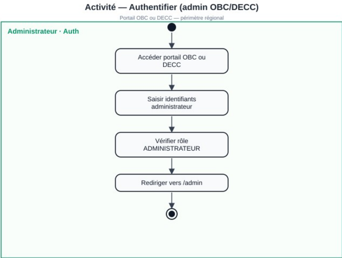
Figure 3.21 — Activité : authentification admin
