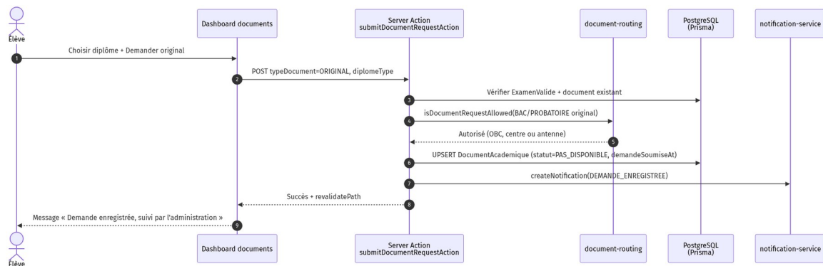
Figure 3.13 — SEQ-ELEVE-04 : demande diplôme original *(variante routage)*
