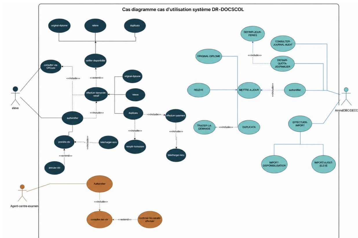
Figure 3.0 — Diagramme général des cas d'utilisation
