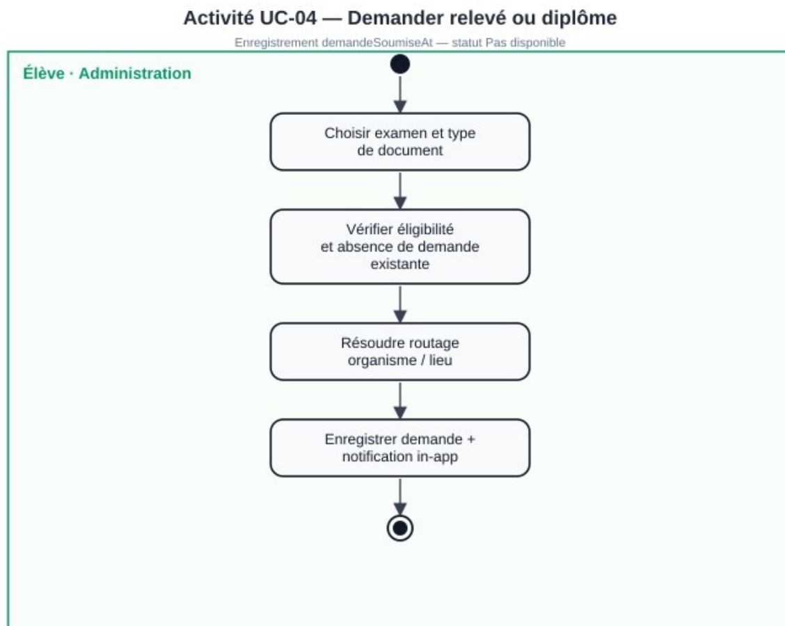
Figure 3.11 — Activité UC-04 : demande relevé / diplôme
