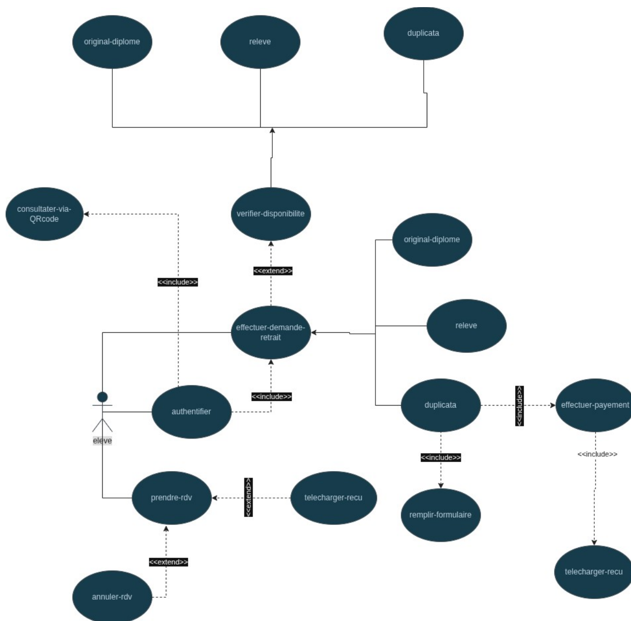
Figure 3.1 — Diagramme de cas d'utilisation — package Élève
