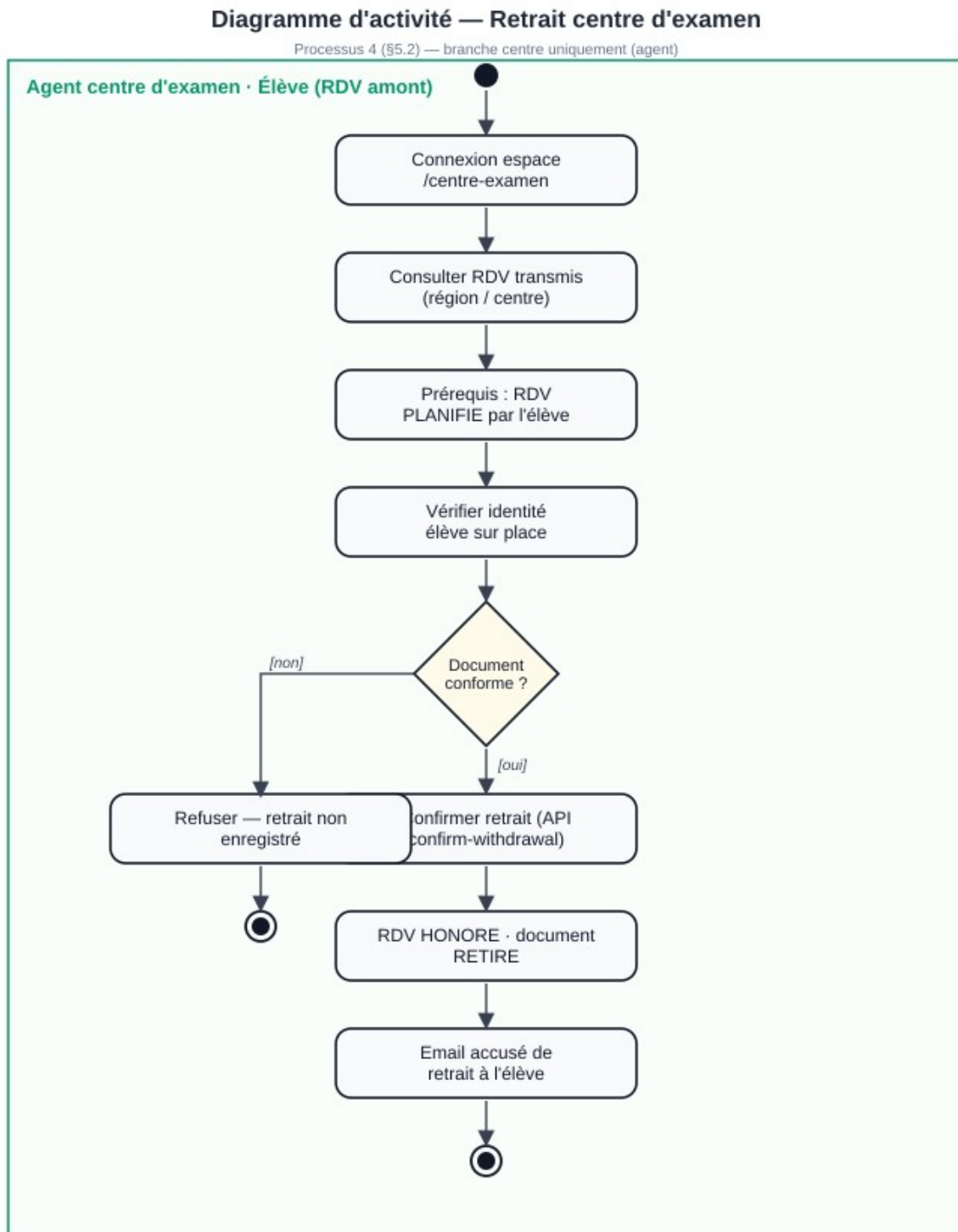
Figure 3.36 — Activité UC-11b / confirmation retrait (ACT-04)
