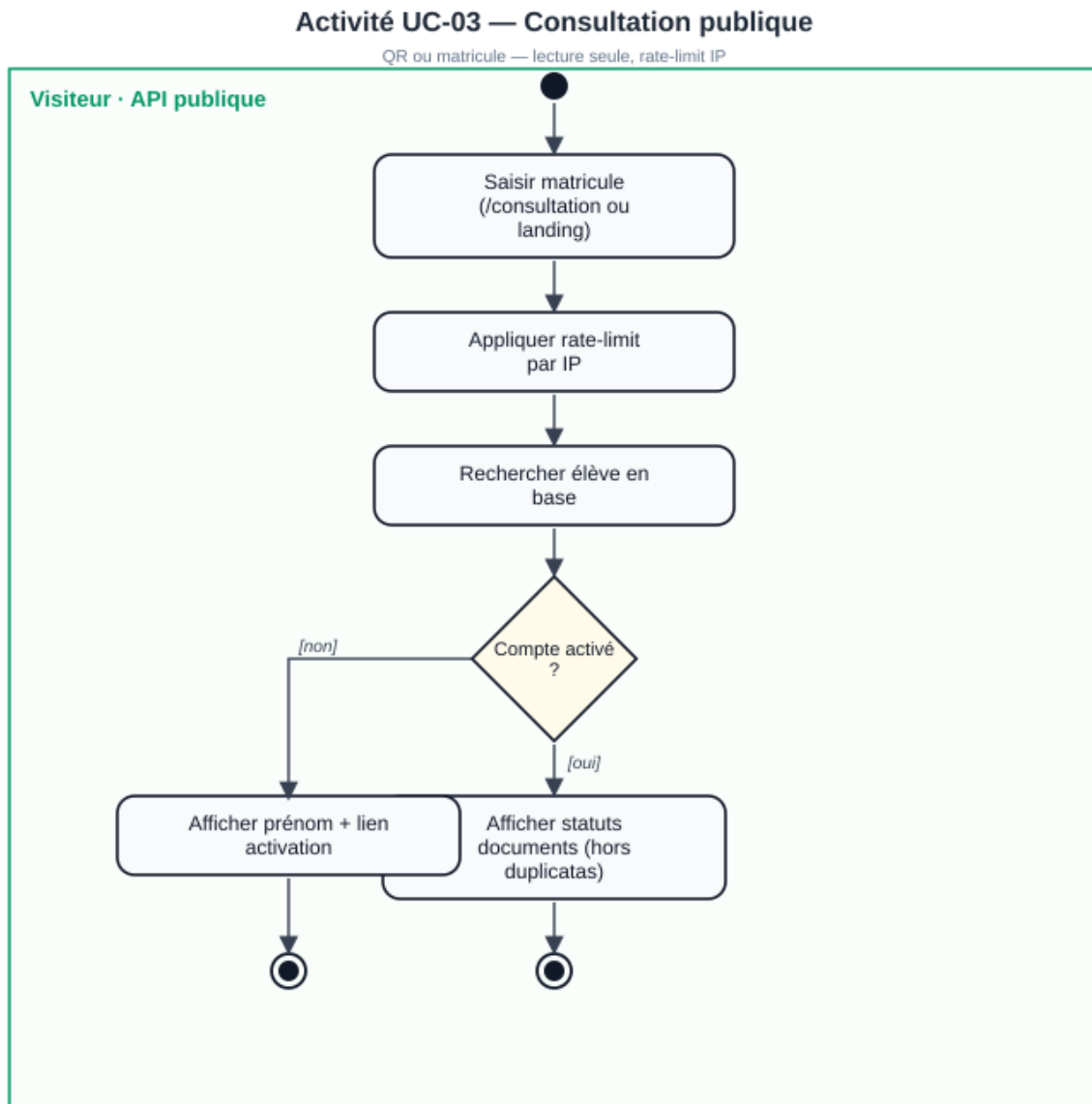
Figure 3.7 — Activité UC-03 : consultation publique
