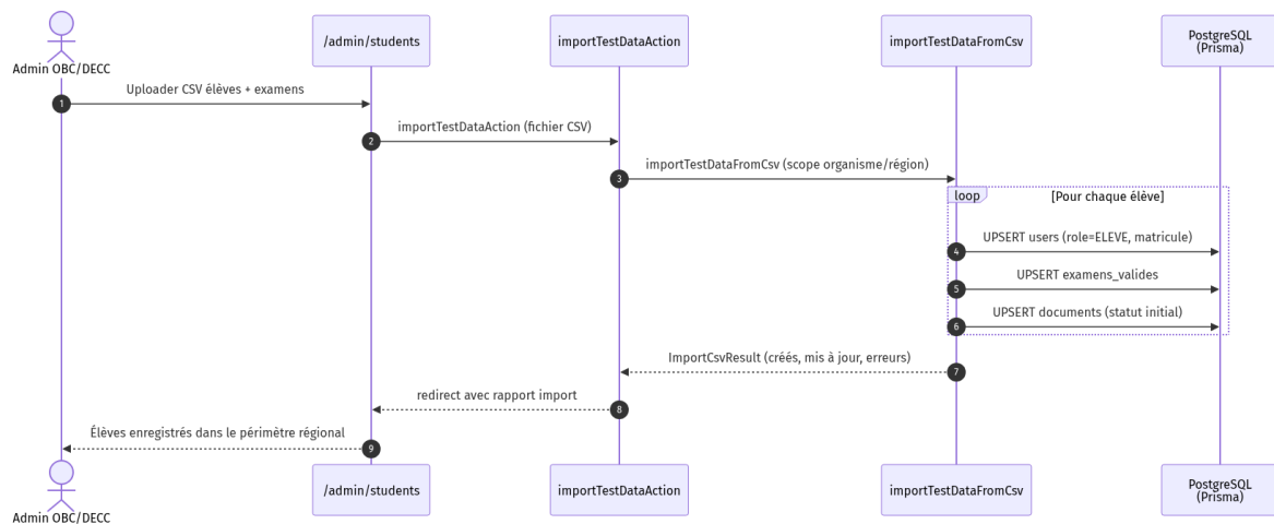
Figure 3.24 — SEQ-ADMIN-11 : import élèves CSV
