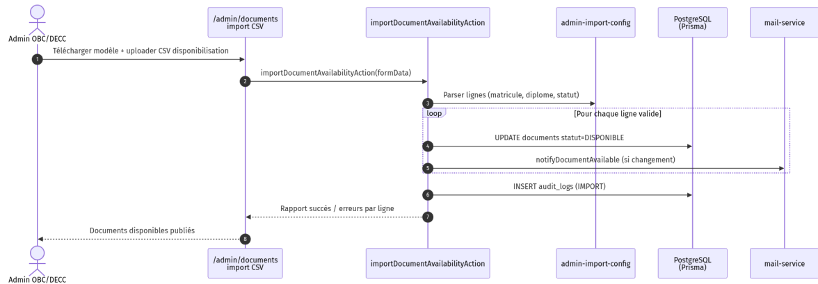
Figure 3.26 — SEQ-ADMIN-10 : import disponibilisation
