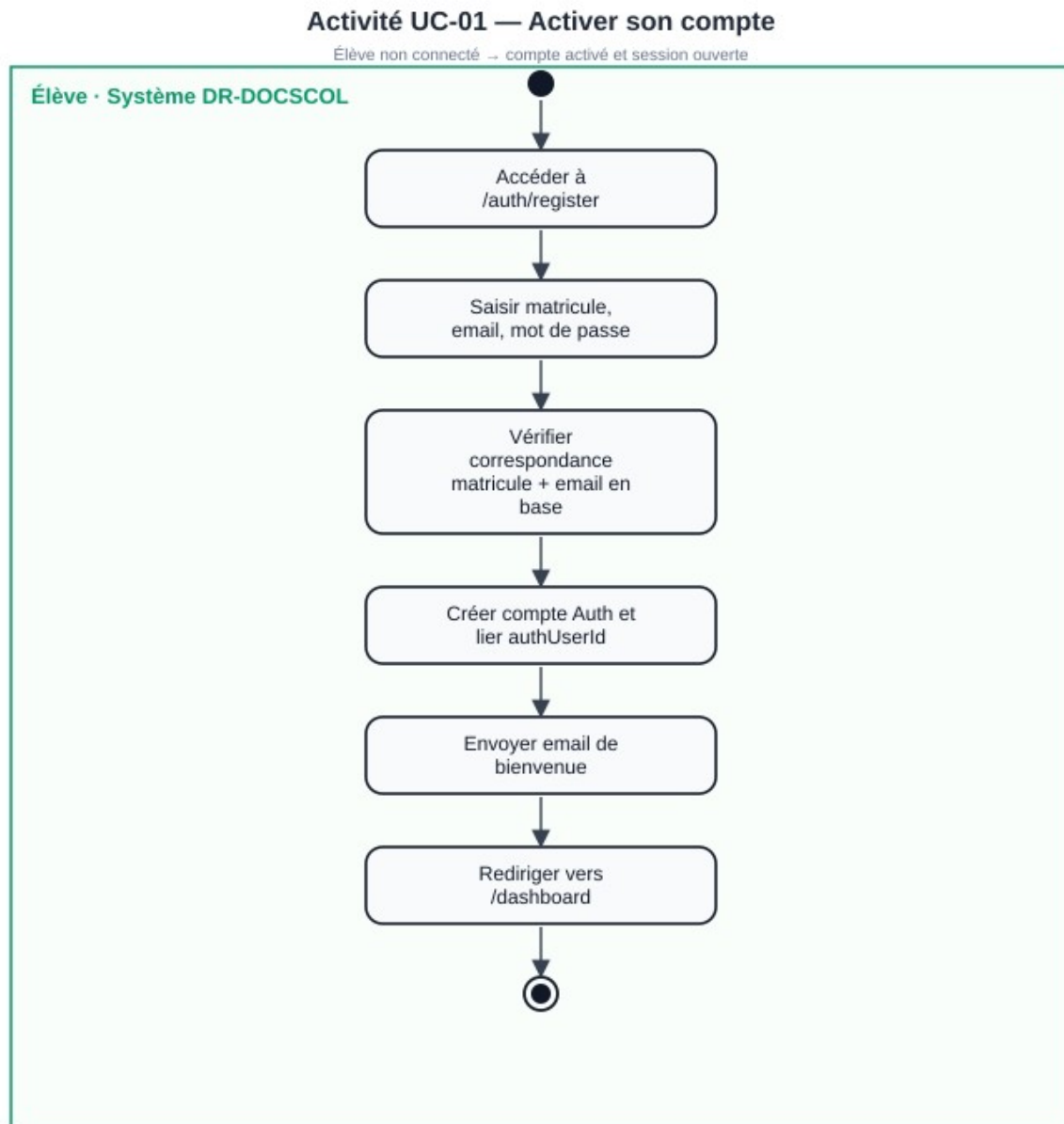
Figure 3.4 — Activité UC-01 : activation de compte
