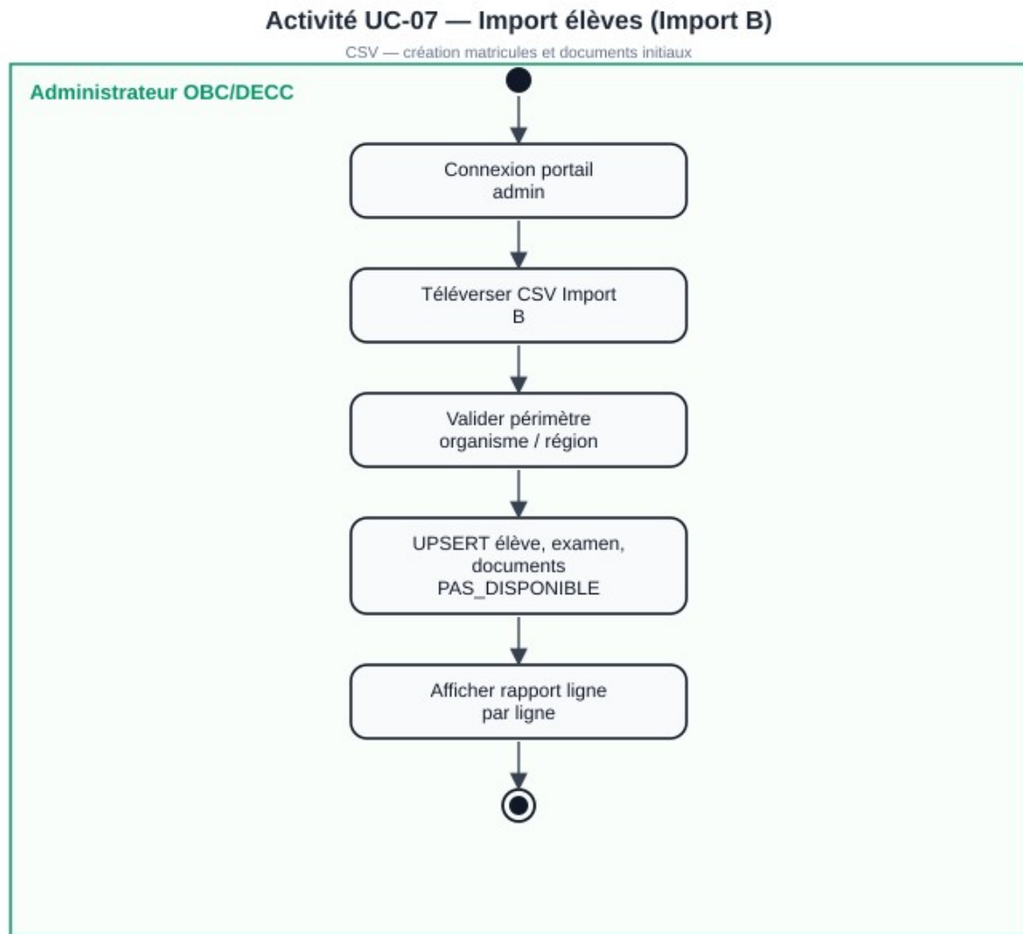
Figure 3.23 — Activité UC-07 : Import B
