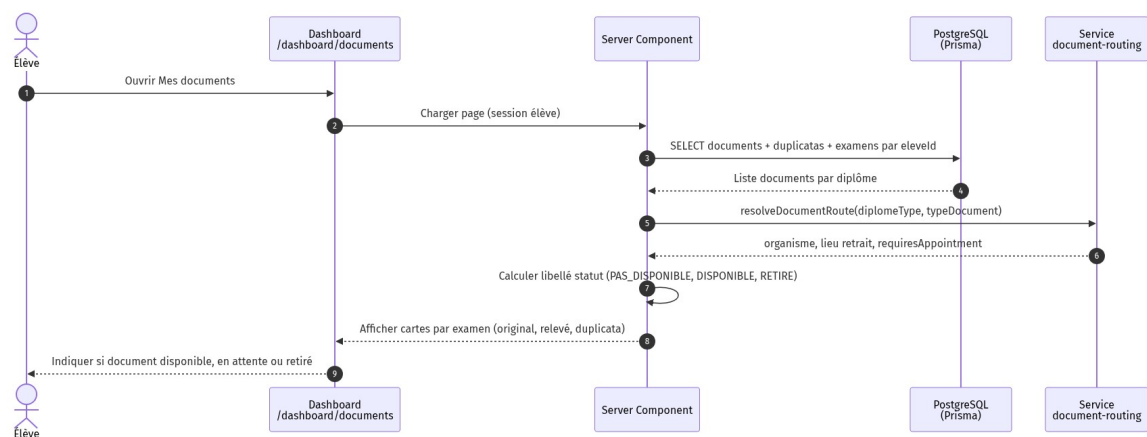
Figure 3.10 — SEQ-ELEVE-03 : vérifier disponibilité
