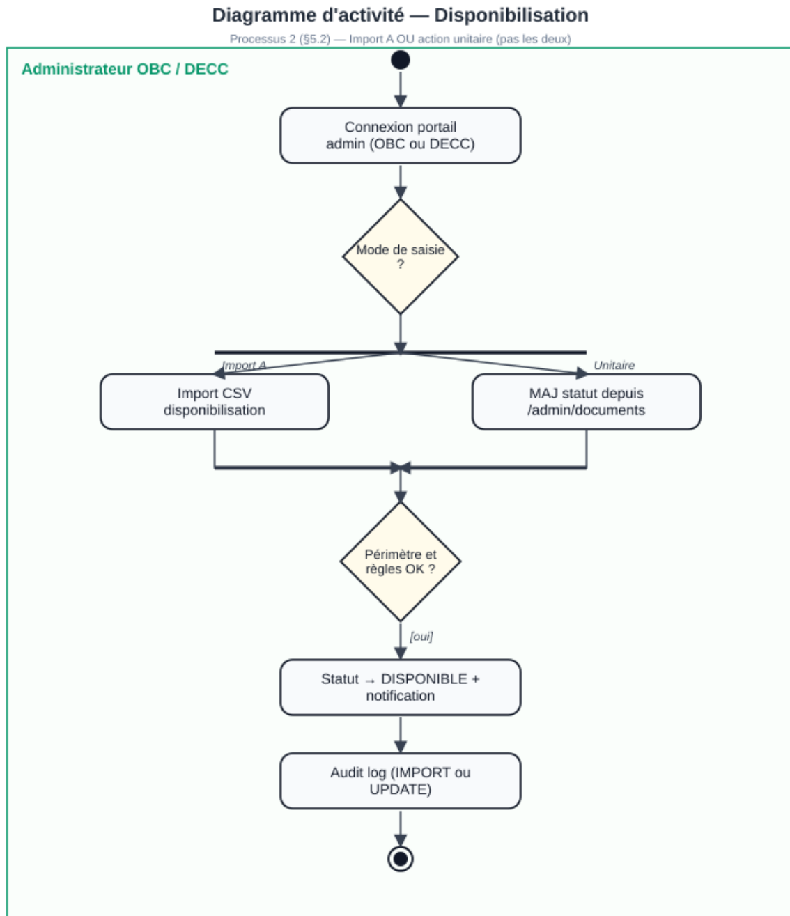
Figure 3.25 — Activité UC-08 / disponibilisation (ACT-03)
