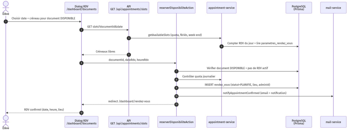
Figure 3.19 — SEQ-ELEVE-09 : prise de rendez-vous
