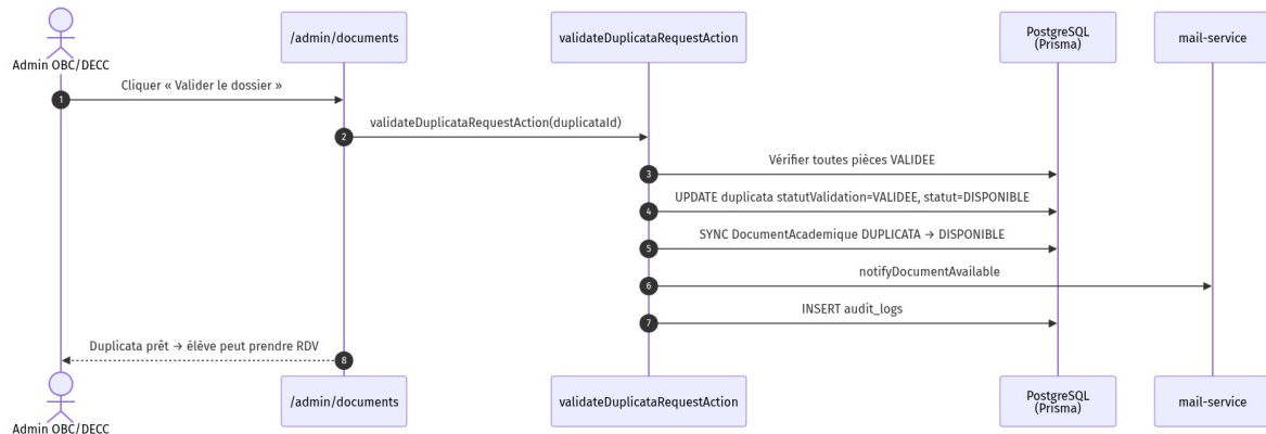
Figure 3.30 — SEQ-ADMIN-08 : valider demande duplicata
