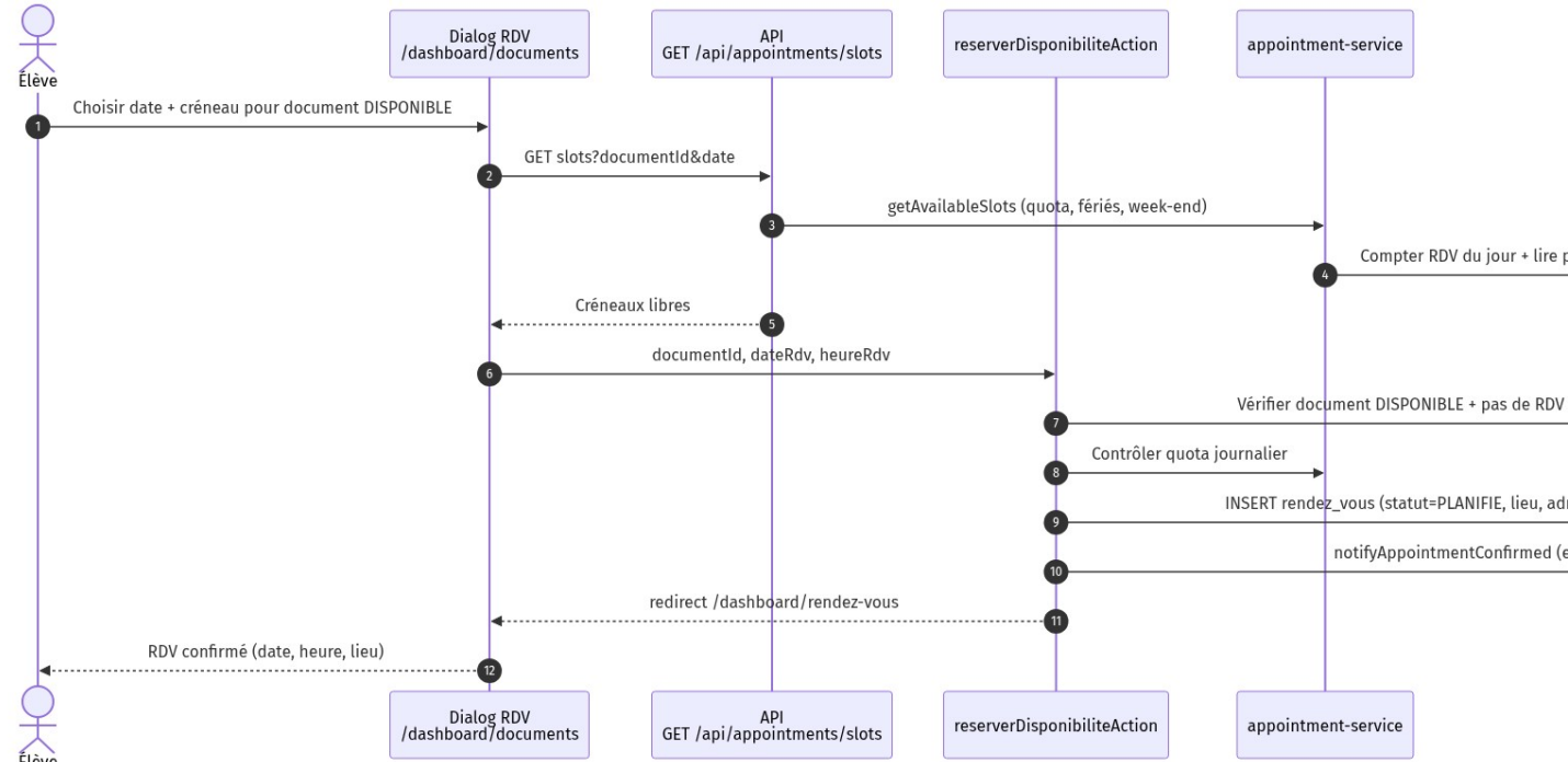
Figure 3.19 — Séquence prise RDV
