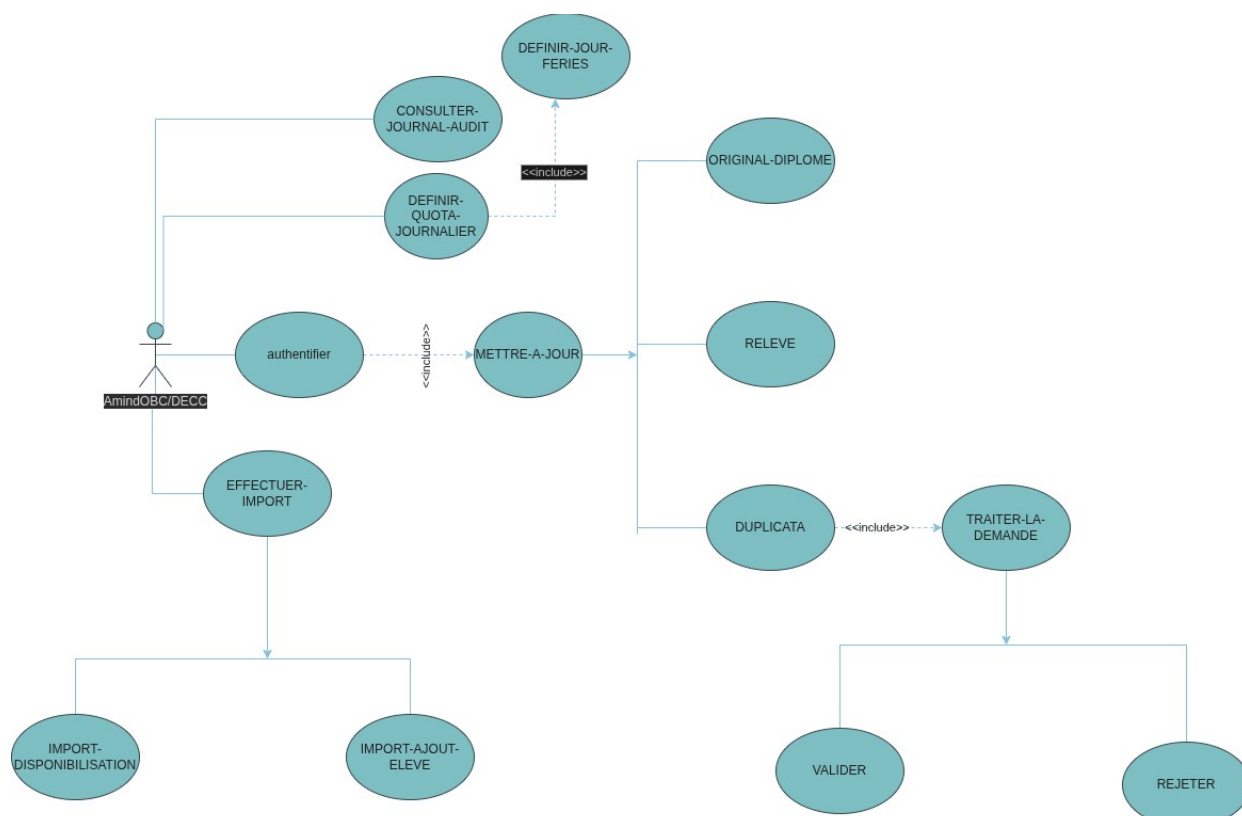
Figure 8.9 — Diagramme de cas d'utilisation — Module Administrateur
