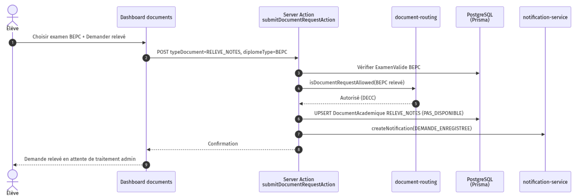
Figure 8.5 — SEQ-ELEVE-05 : demande relevé
