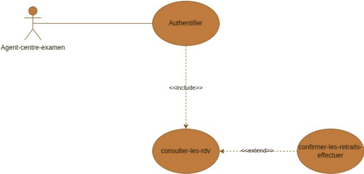
Figure 8.15 — Diagramme de cas d'utilisation — Module Agent centre
