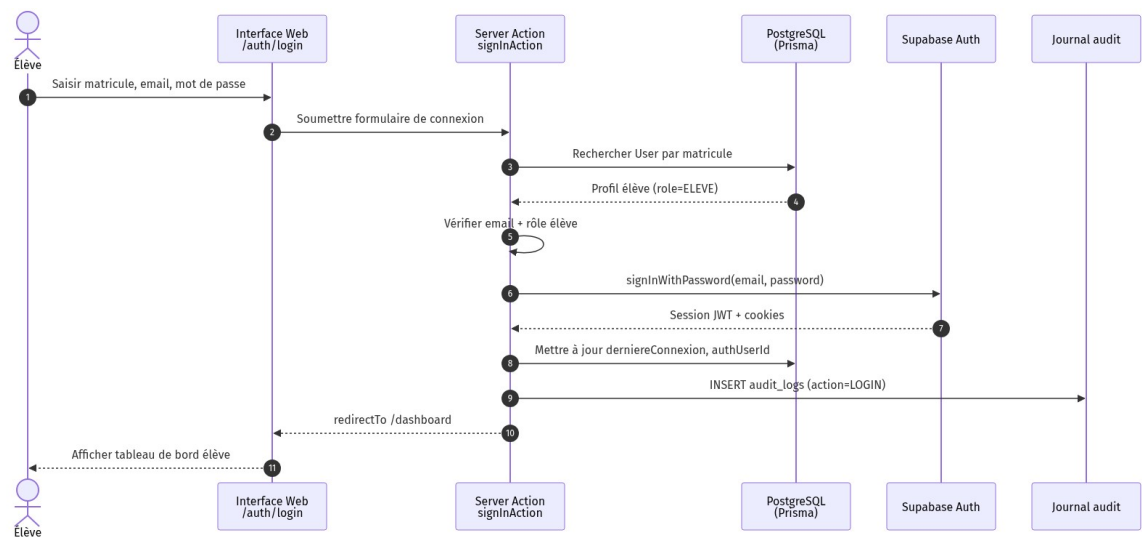
Figure 8.3 — SEQ-ELEVE-01 : authentification élève
