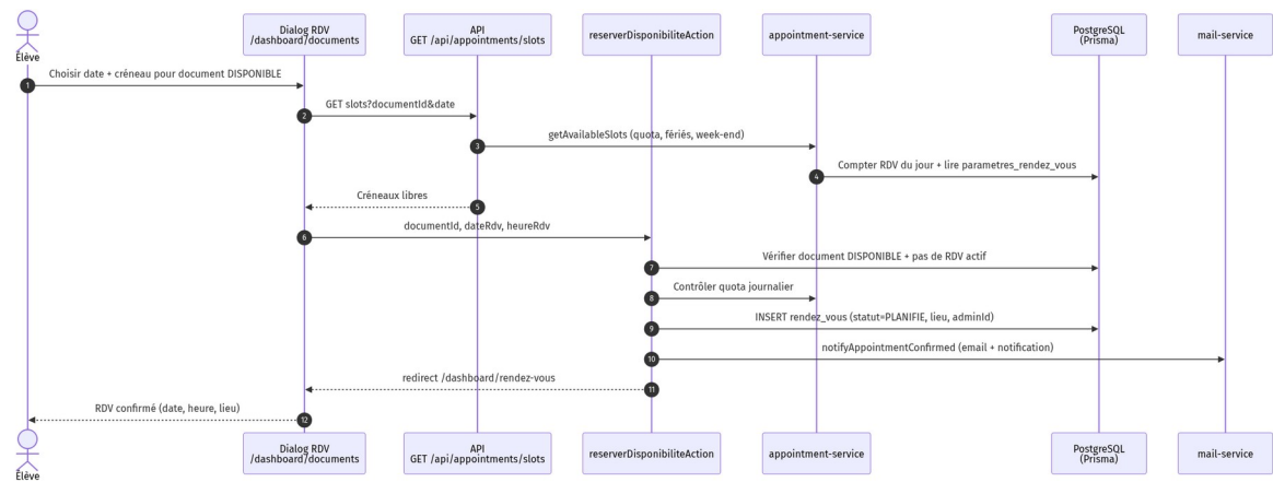
Figure 8.8 — SEQ-ELEVE-09 : prise de rendez-vous
