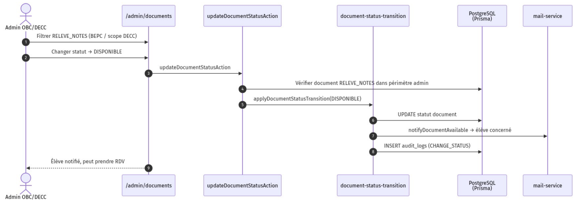
Figure 8.14 — SEQ-ADMIN-06 : mise à jour statut relevé
