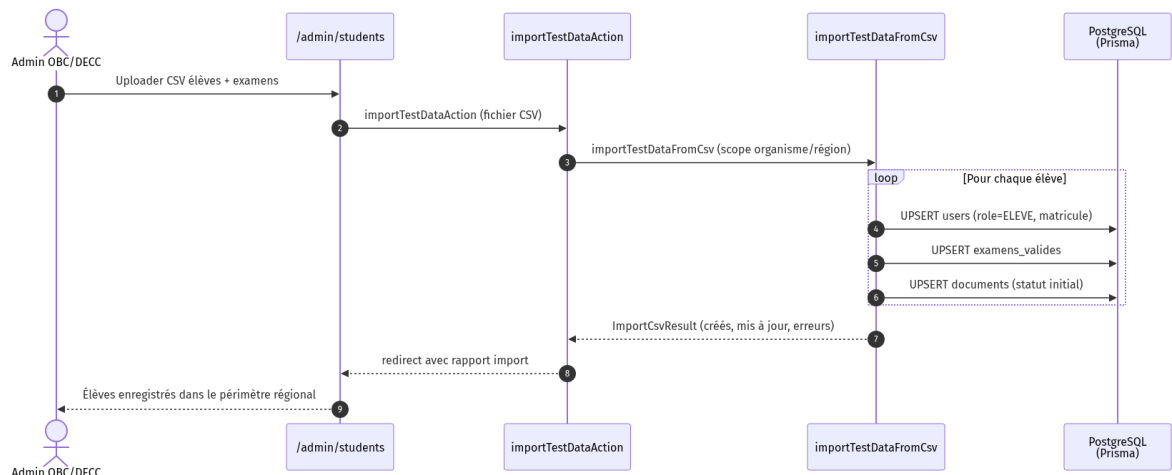
Figure 8.12 — SEQ-ADMIN-11 : import élèves
