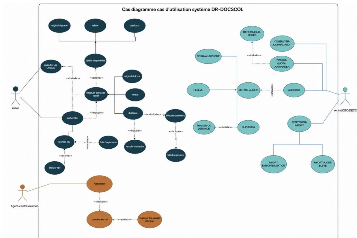
Figure 8.1 — Diagramme général (trois acteurs)
