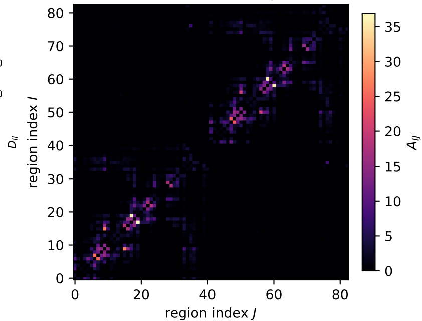
(c) Adjacency A_{IJ}
