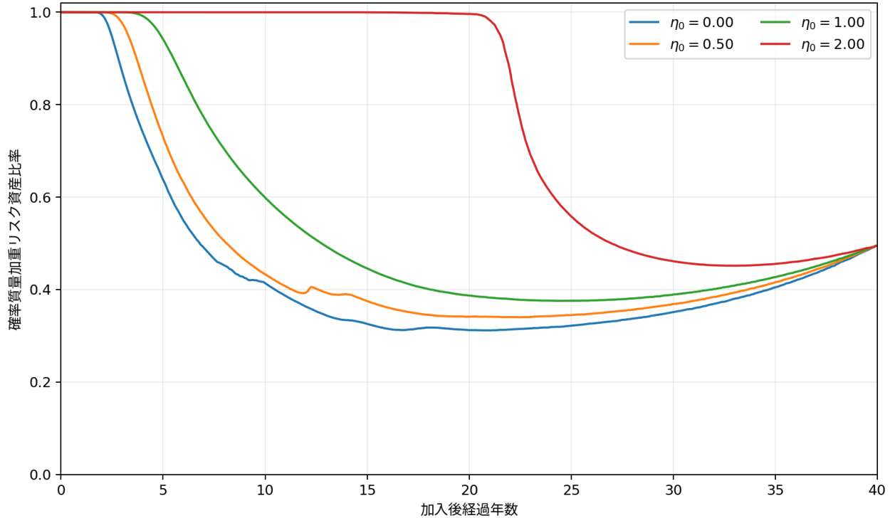
図 7: dTCMV-MVS の係数別グライドパス. 分散回避係数を \gamma_0 = 2.5 に固定し、歪度係数を \eta_0 = 0, 0.5, 1.0, 2.0 とした。各曲線は、各方針が生成する前進分布で加重したリスク資産比率である。
