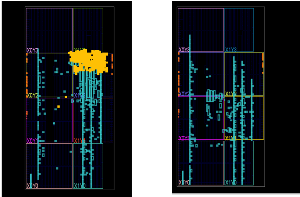
איור 19: מפת המשאבים על גבי הסיליקון: מימין המערכת ללא ILA, ומשמאל תוספת החומרה עבור מערכת הדיבוג
