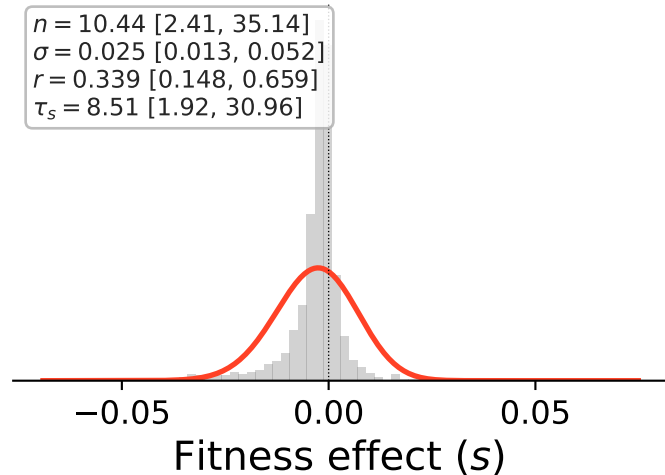
MNO R
