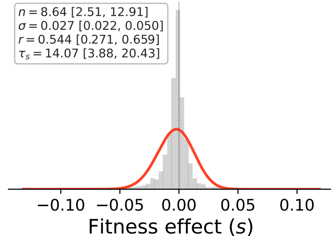
REL607 (2)
