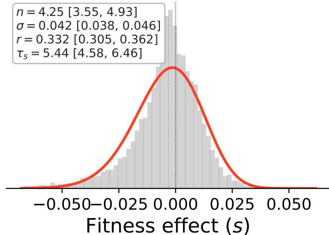
REL607 (1)
