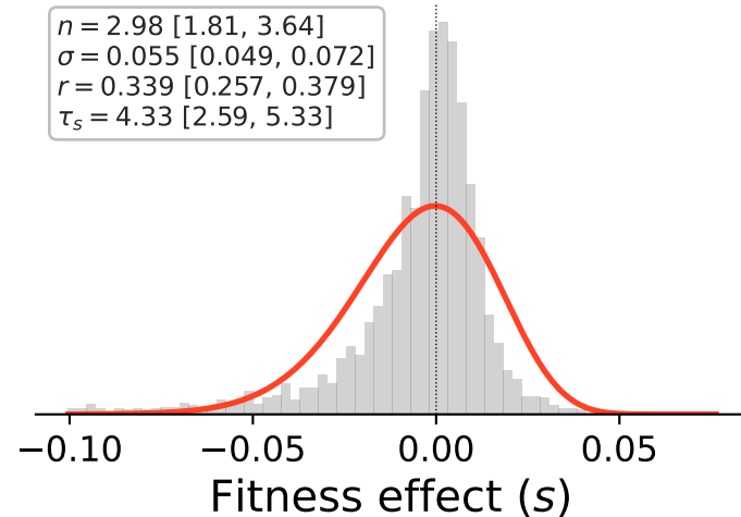
REL607 (2)
