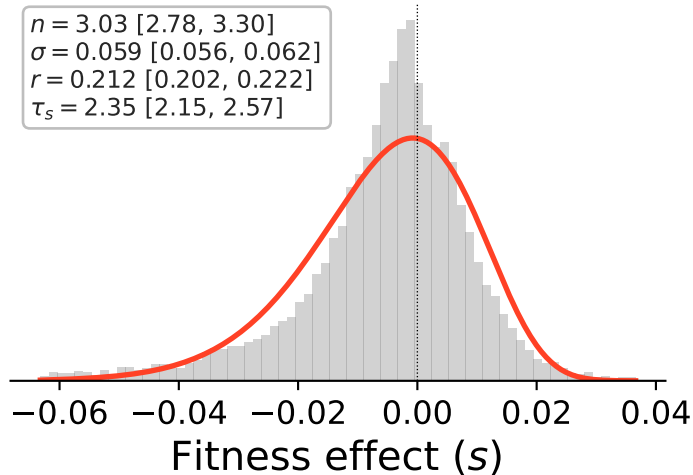
ARA+2 (2K)
