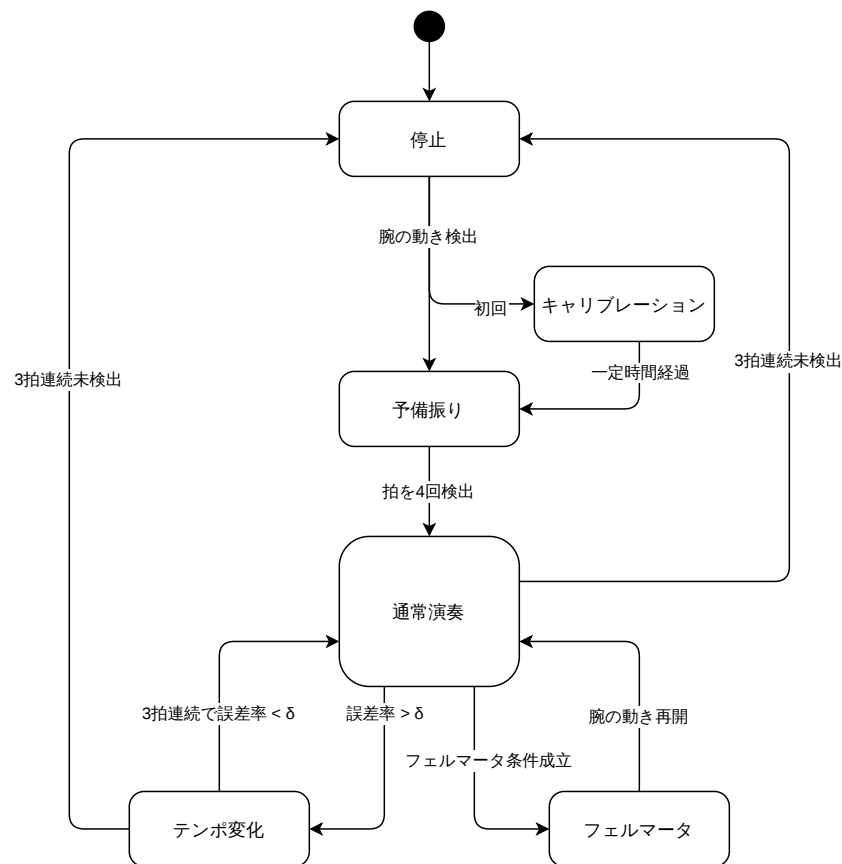
図 2.5 状態遷移図
