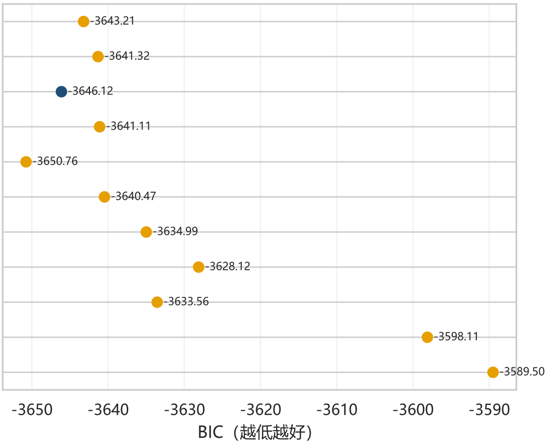
BIC比较
