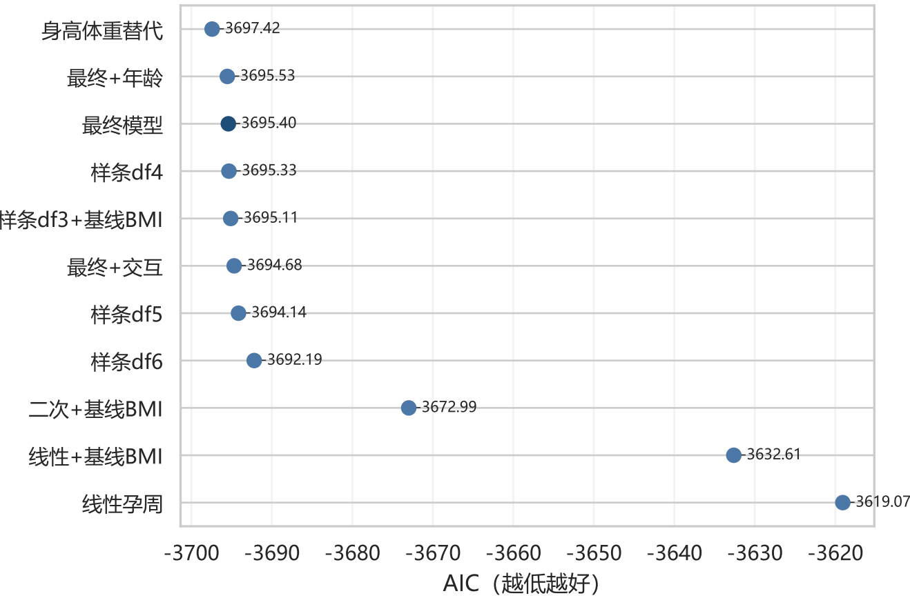
AIC比较
