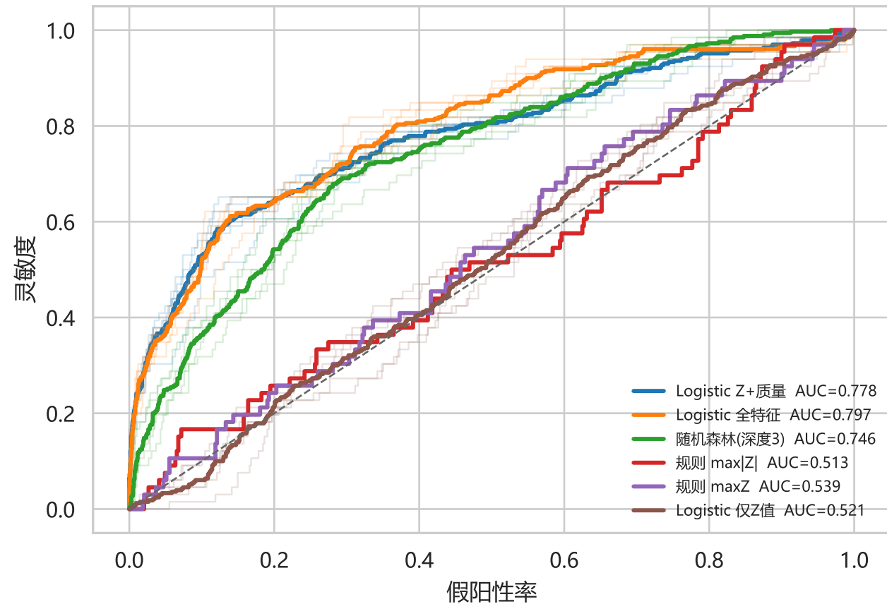
A. ROC 曲线 (细线为各次重复)
