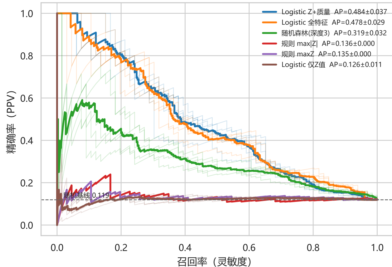
B. PR 曲线：类别不平衡下更能反映实际表现
