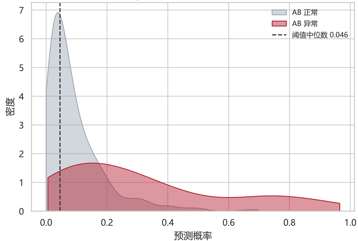
B. Logistic Z+质量 的预测分布与阈值
