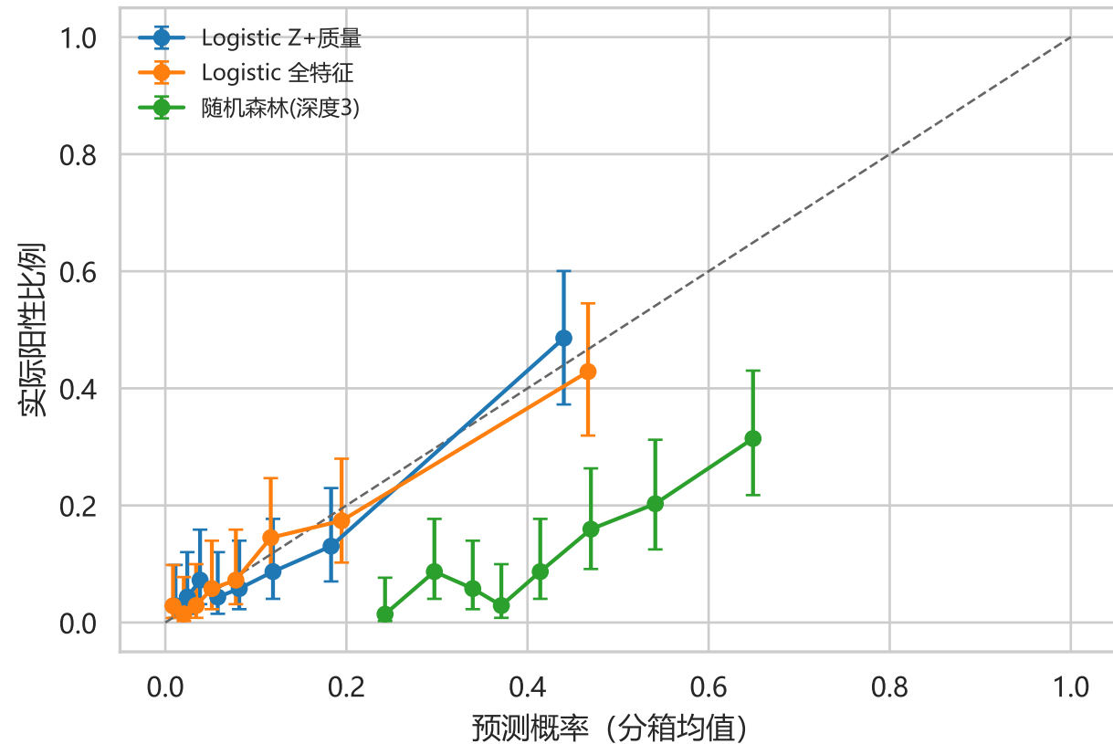
A. 概率校准 (误差棒为 Wilson 95% 区间)
