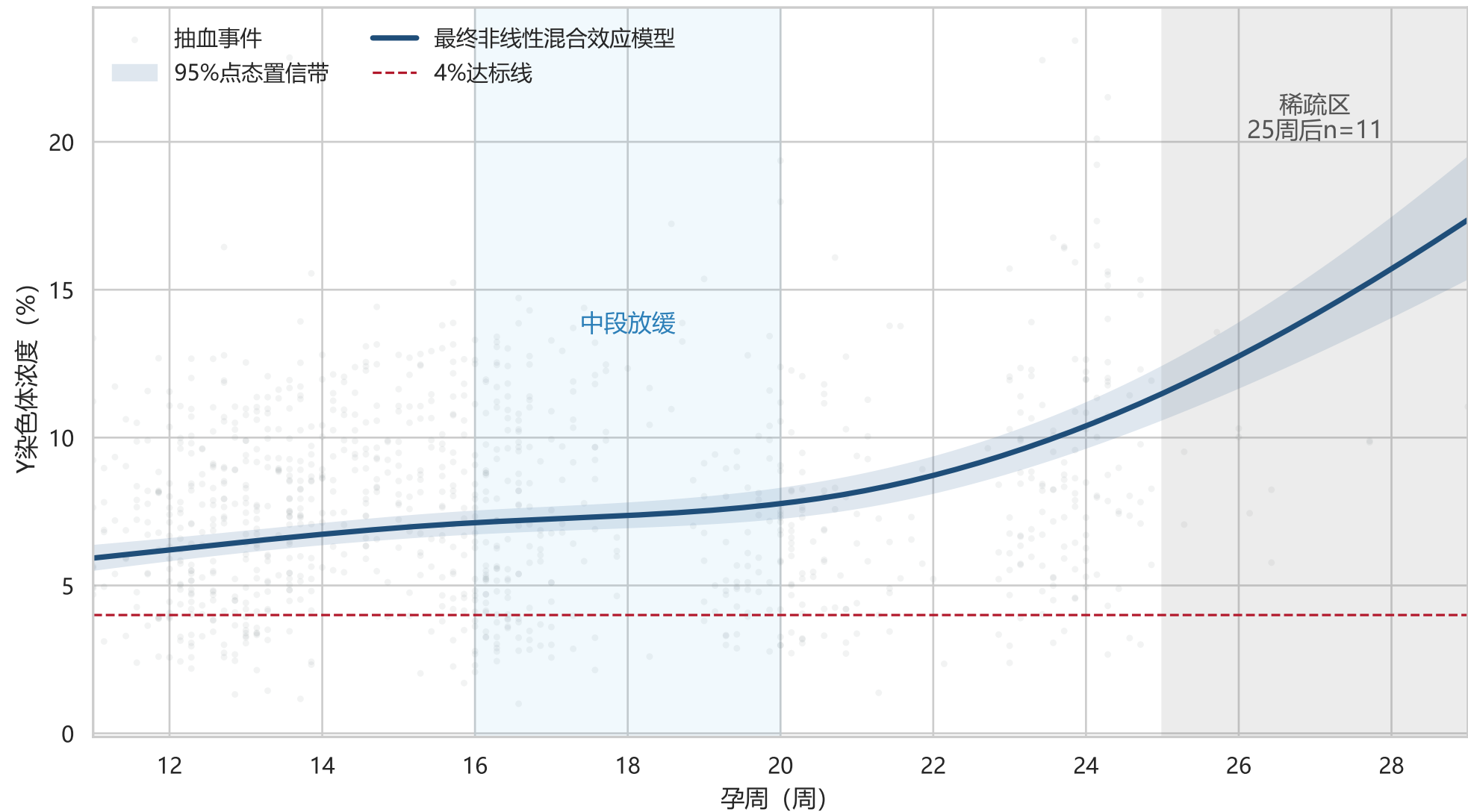
最终非线性混合效应模型的孕周效应
