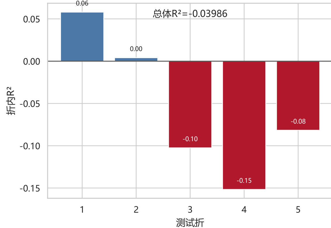
B. 最终模型各折预测R 2
