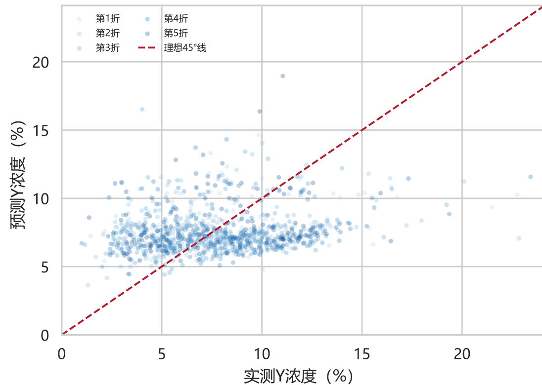
A. 最终模型：新孕妇预测值 vs 实测值
