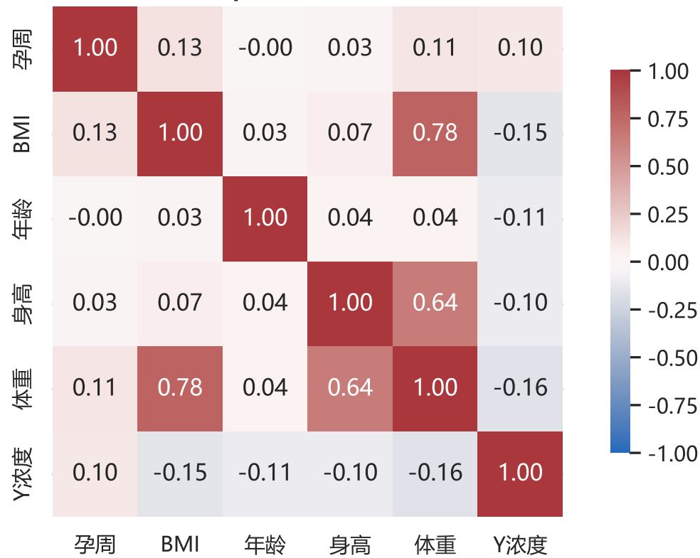
C. 事件级Spearman相关 (描述性)
