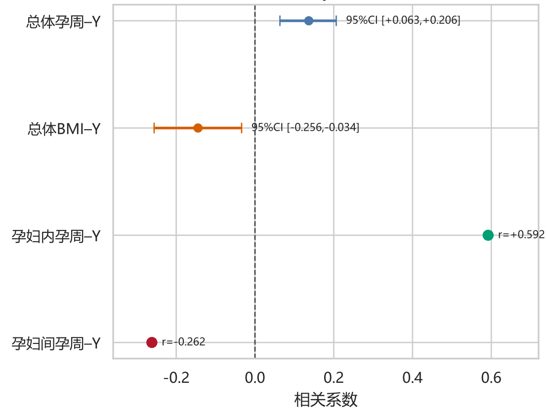
D. 聚类Bootstrap及组内/组间相关
