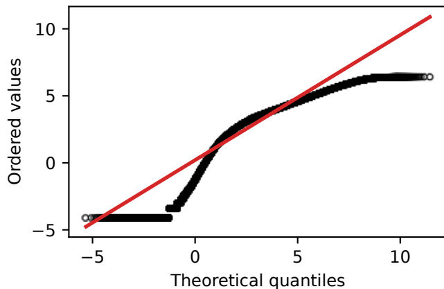
(d) MoreUser: QQ vs Normal
