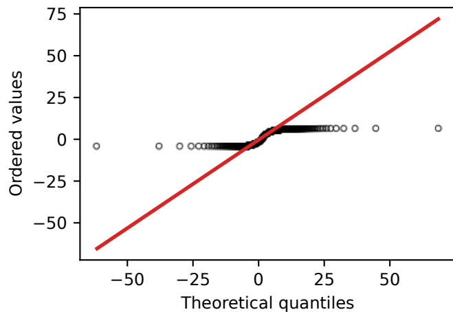
(d) MoreUser: QQ vs Student-t
