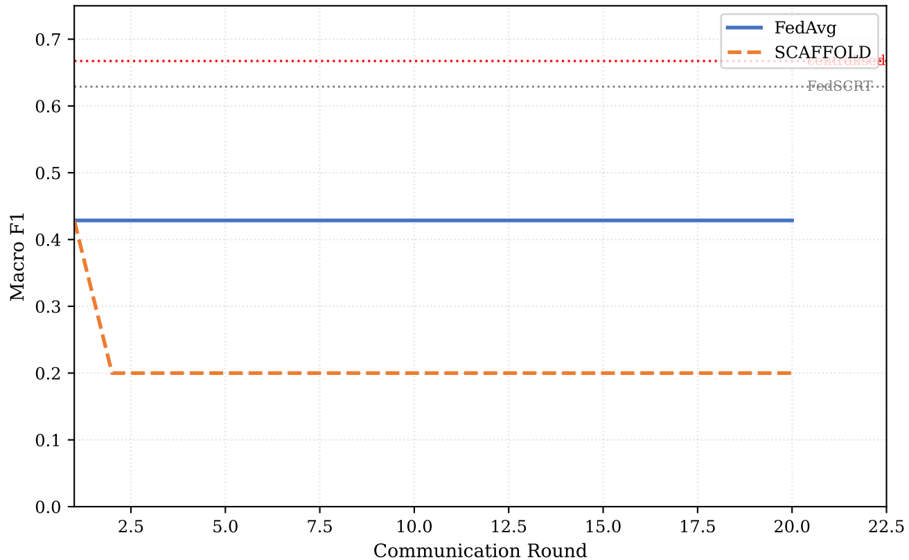
F1 per Communication Round
