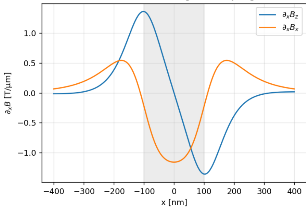
z = -100 \text{ nm} (2DEG) — gradient (jax.grad)
