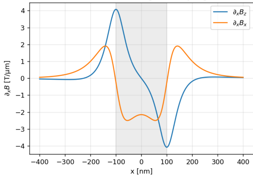
z = -100 \text{ nm} (2DEG) — gradient (jax.grad)
